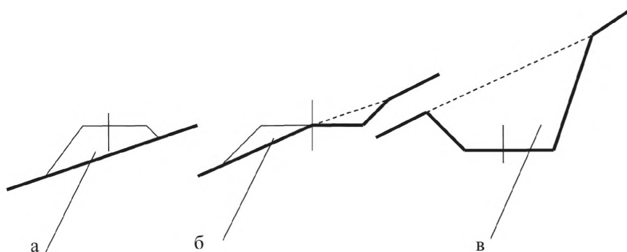
а) насыпь; б) полунасыпь-полувыемка; в) выемка
