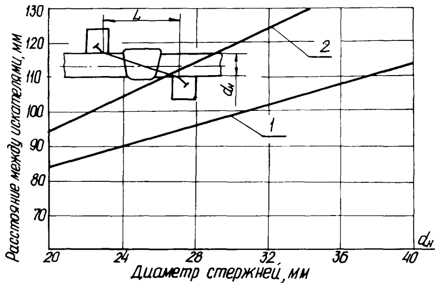
Рис. 4 Графики выбора расстояния между искателями в зависимости от диаметра стержня для способов сверки ВП-Г, ВМ-Г, ВО-Б (кривая 1) и ВП-В (кривая 2) по ГОСТ 14098-68
