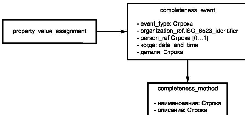
Рисунок 1 — Диаграмма класса UML для завершенности данных
