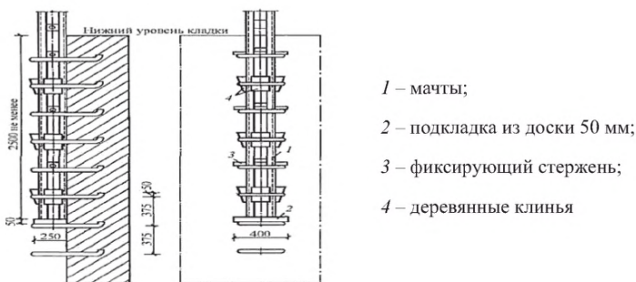
Рисунок 13 – Крепление мачты крана-укосины в скобах
