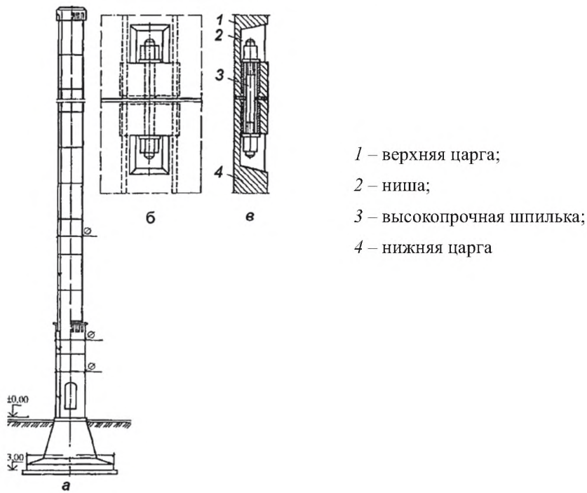
а – общий вид; б, в – узлы крепления
