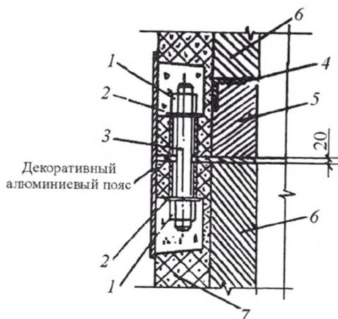
1 – гайка; 2 – шайба; 3 – шпилька; 4 – уголок, приваренный к закладной детали царги; 5 – футеровка после монтажа; 6 – домонтажная; 7 – царга
