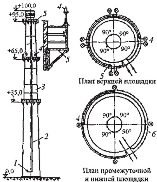
Рисунок Б.1 – Светограждение трубы
