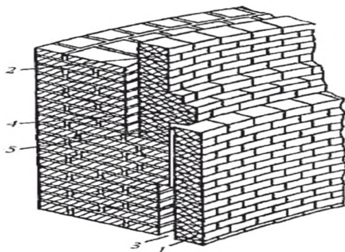
1 – нижнее звено футеровки; 2 – верхнее звено футеровки; 3 – воздушный зазор; 4 – температурный зазор; 5 – ствол трубы
