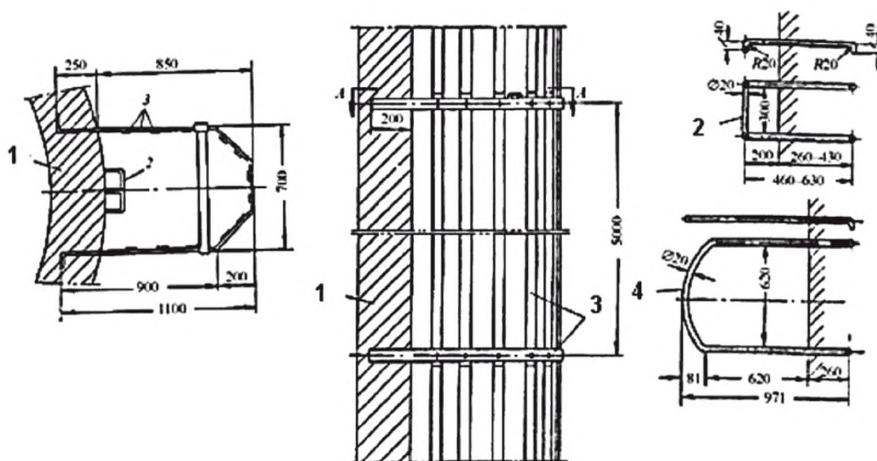
1 – ствол трубы; 2 – ходовые скобы; 3 – ограждение скоб; 4 – скоба для отдыха
