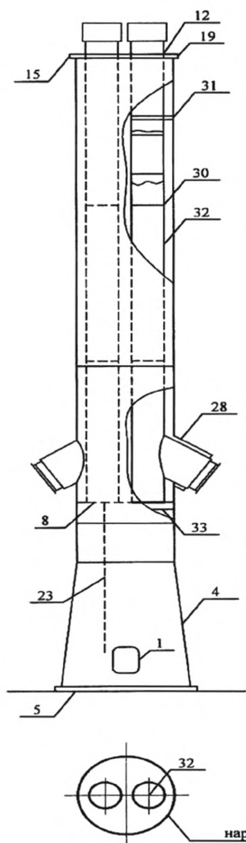
Рисунок Б.3 – Самонесущая многоствольная труба
