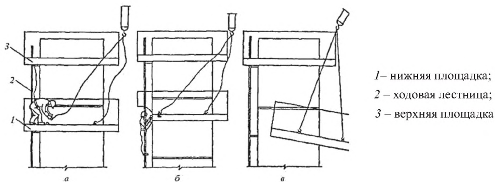
а – закрепление стропа, б – разбалчивание соединительной шпильки, в – спуск площадки на землю
