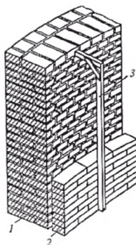
Рисунок 16 – Проверка уклона футеровки
