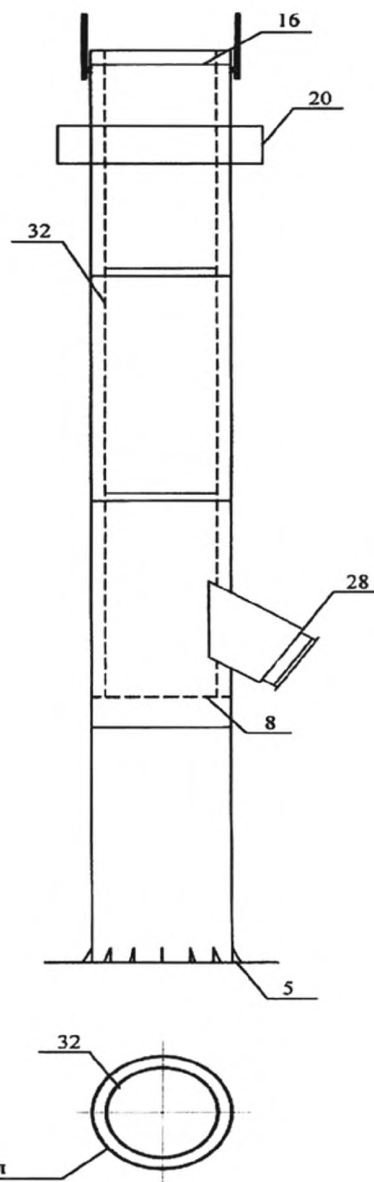
Рисунок Б.4 – Труба с двойной стенкой
