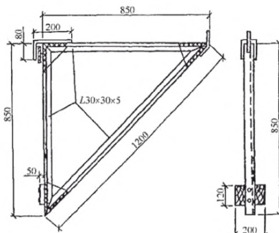
Рисунок 14 – Металлический кронштейн
