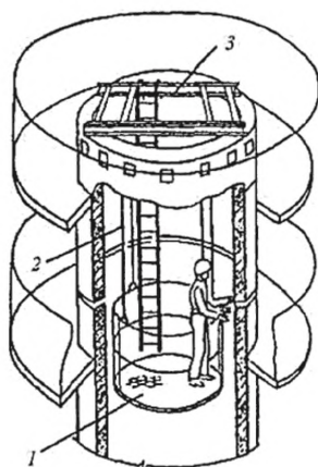
1 – площадка; 2 – тяга; 3 – опорная рама
