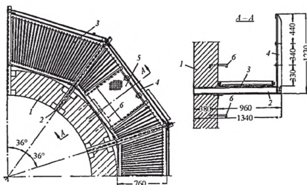
Рисунок 4 – Замок стяжного кольца
