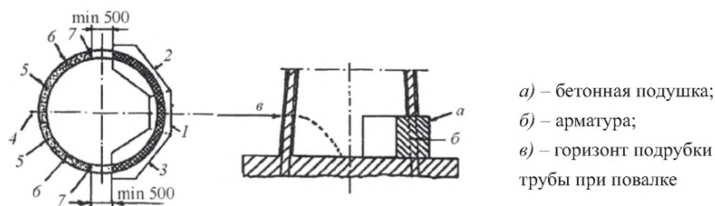
1 – начальный сегмент вырубki ствола; 2,3 – последующие сегменты; 4, 5, 6, 7 – очередность подрубки ствола после устройства бетонной подушки
