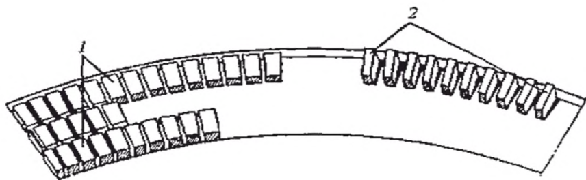
1 – кирпич, уложенный на растворе; 2 – накерстанный кирпич
