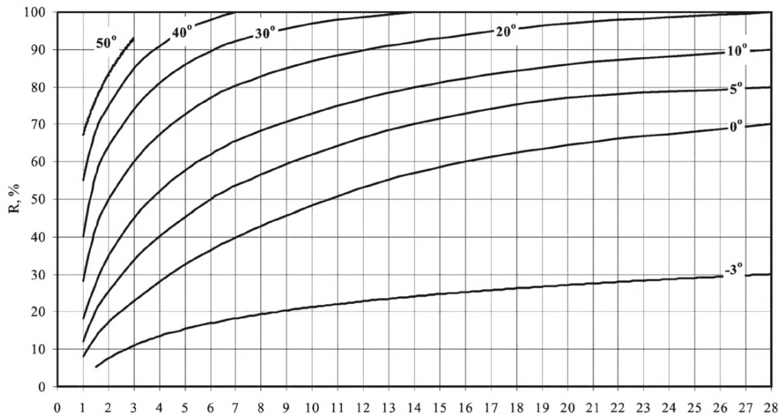
Рисунок 20 – График нарастания прочности бетона класса В30 на портландцементе марки 400
