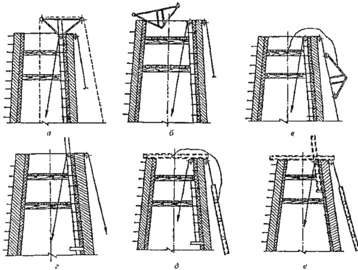
a – спуск мачты до уровня касания оголовка обреза кладки; б – демонтаж оголовка; в – спуск оголовка на землю; г – подъем мачты до уровня размещения соединительного фланца выше рабочего настила; д – разборка мачты и опускание верхней ее части на землю; е – подъем нижней части мачты в скобах и спуск ее на землю
