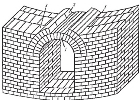
Рисунок 11 – Кладка надземного ввода
