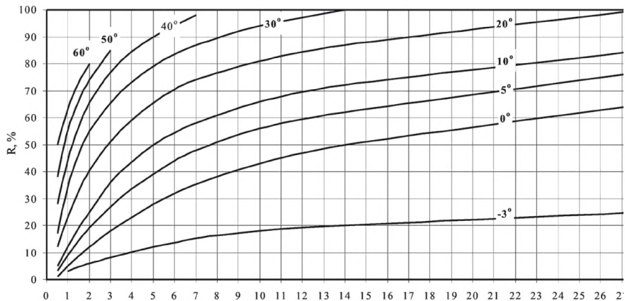
Рисунок 19 – График нарастания прочности бетона классов В15 – В25 на портландцементе марки 400
