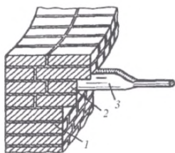
Рисунок 12 – Кладка карниза
