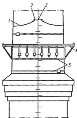
Рисунок 15 – Закрепление обводного каната на трубе
