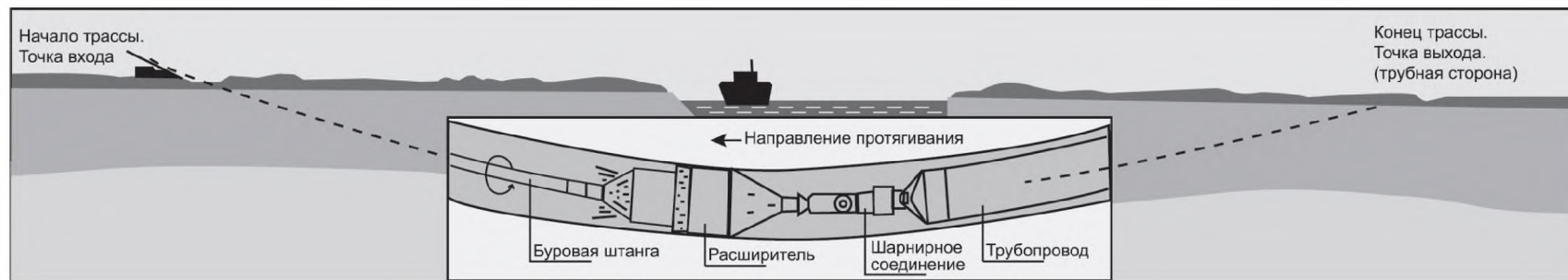
Рисунок 8.7 – Протягивание трубопровода через буровой канал на буровую установку
