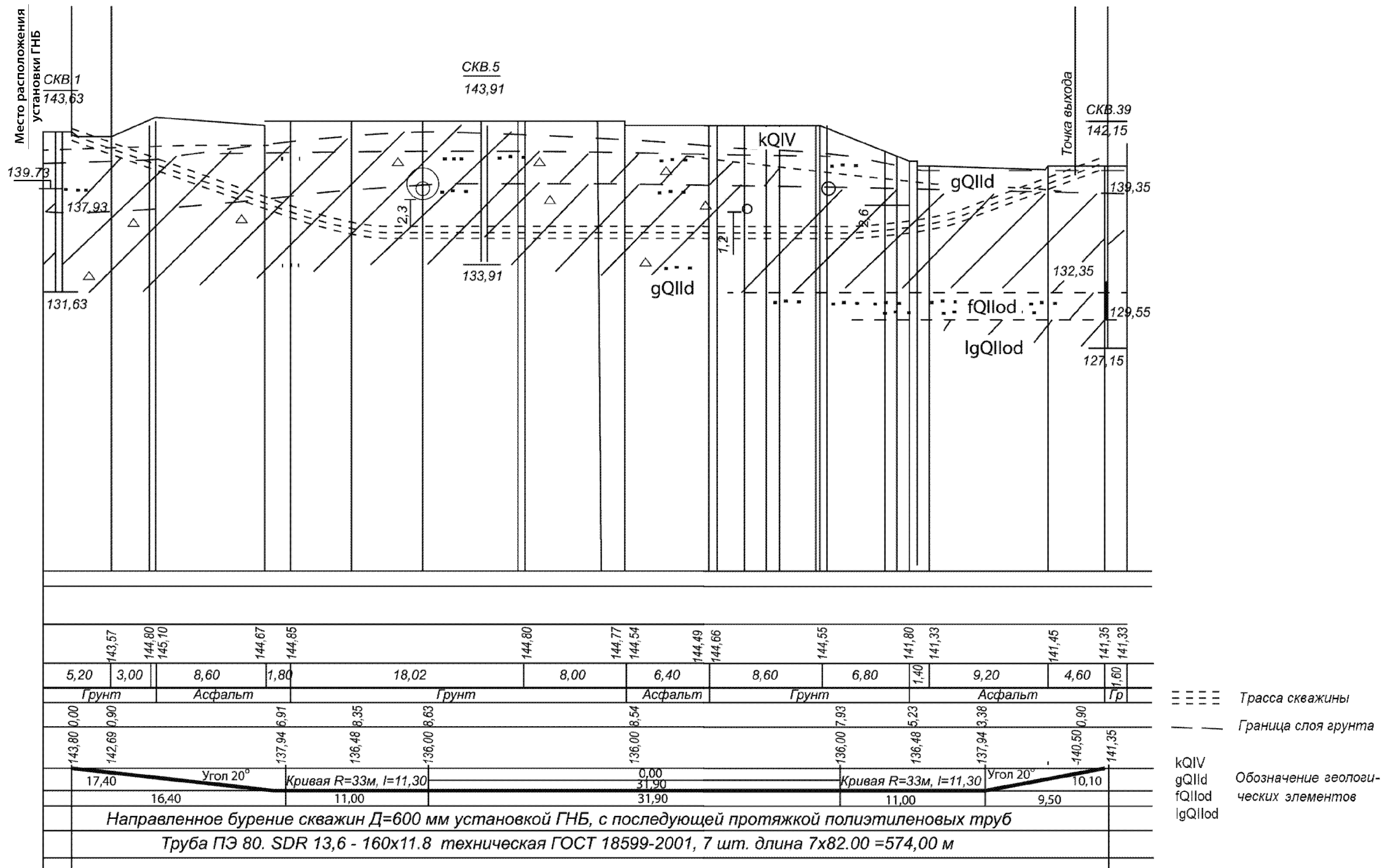
7.1 – Пример построения продольного профиля трассы скважины ГНБ
