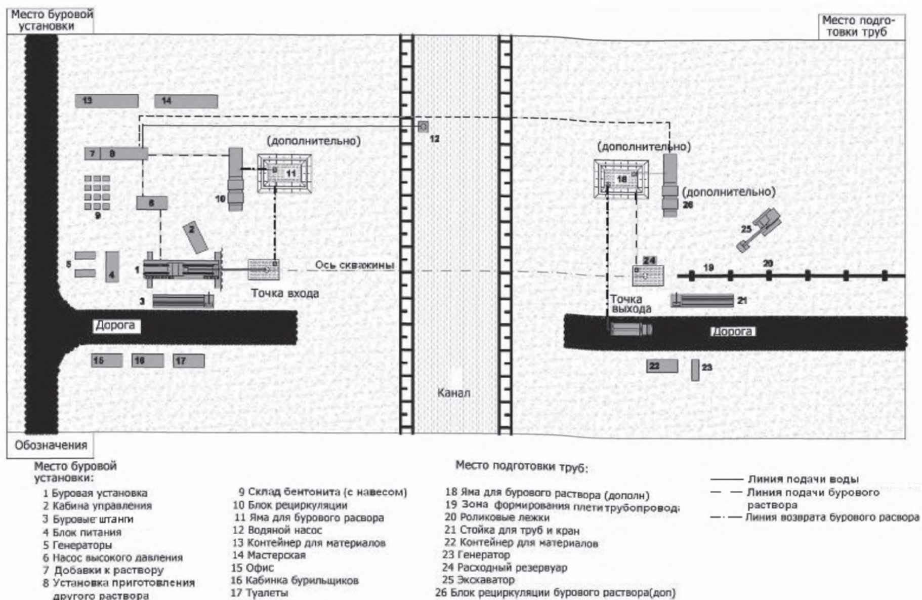
Рисунок 8.1 – Схема расположения оборудования на стройплощадках
