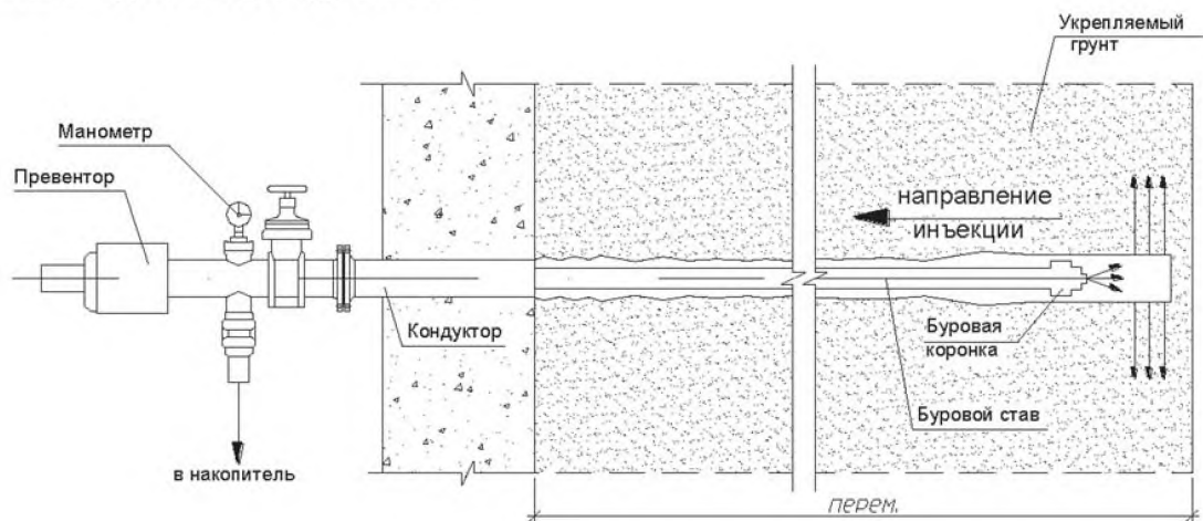
б) инъекция грунтов через буровой став
