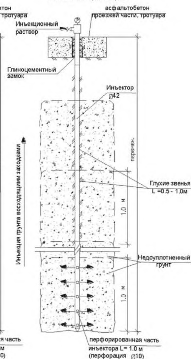
б) Инъекция грунтов силикатным раствором
