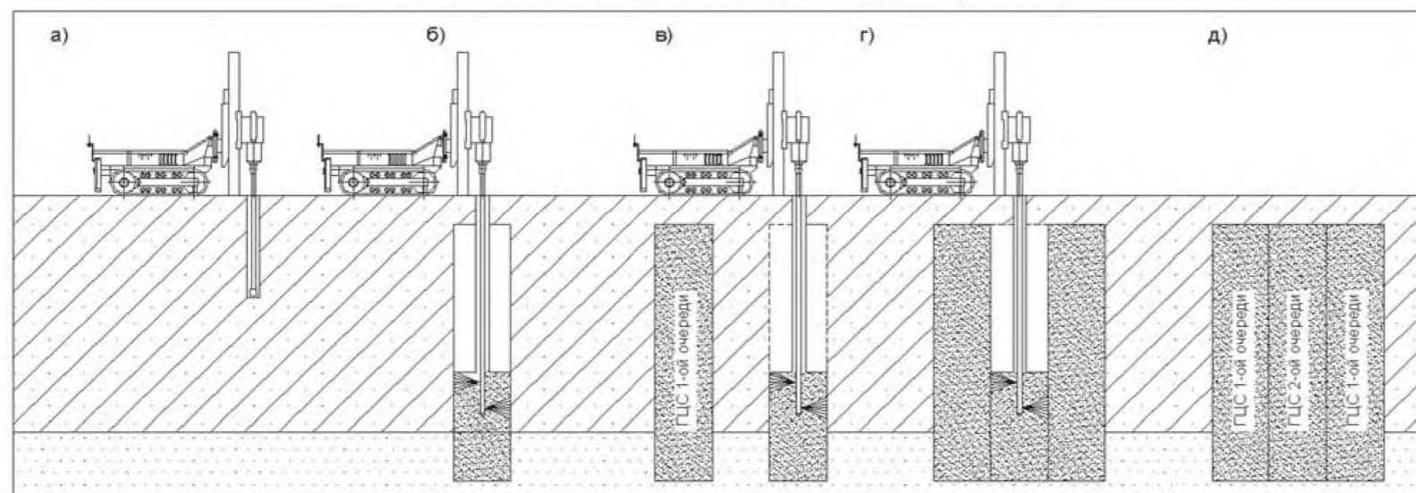
Технология стабилизации грунтов методом струйной цементации
