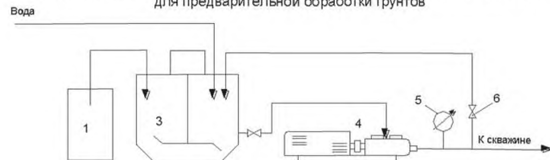
Приготовление и нагнетание активирующего раствора щавелевой кислоты для предварительной обработки грунтов
