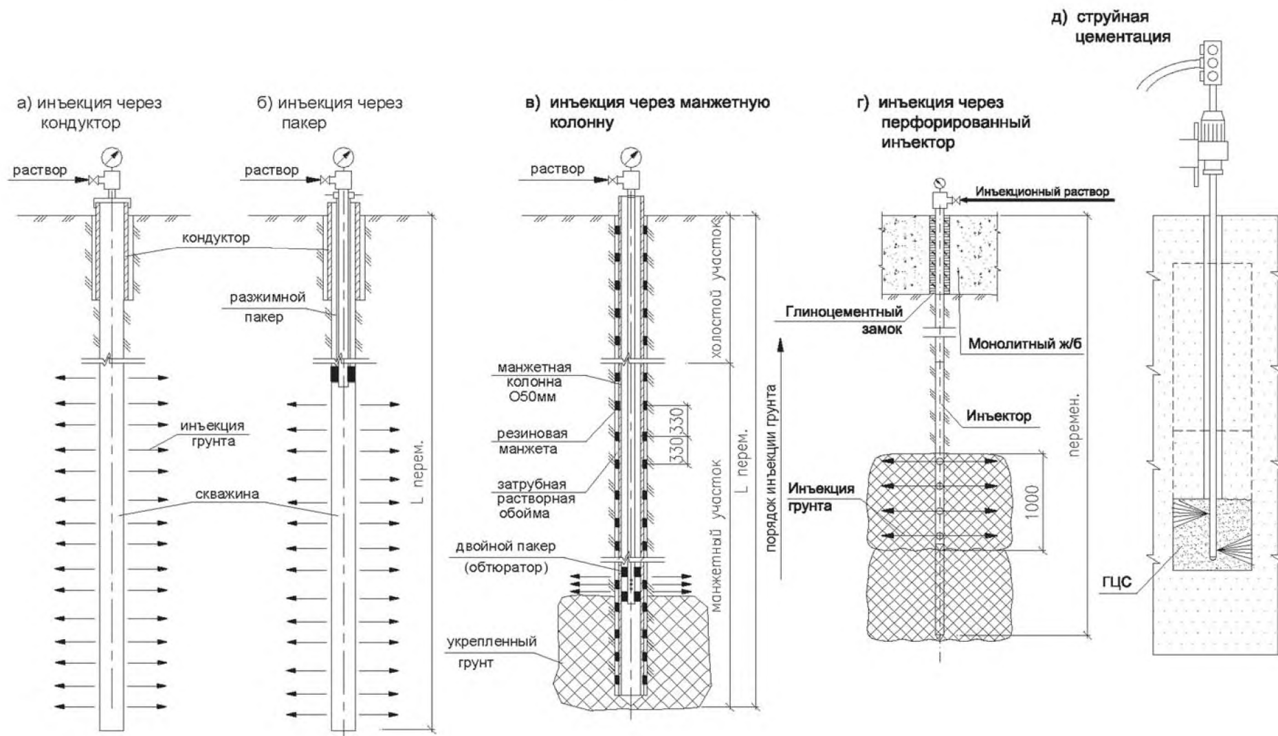
Рисунок В.1 – Оборудование скважин и способы иньекции
