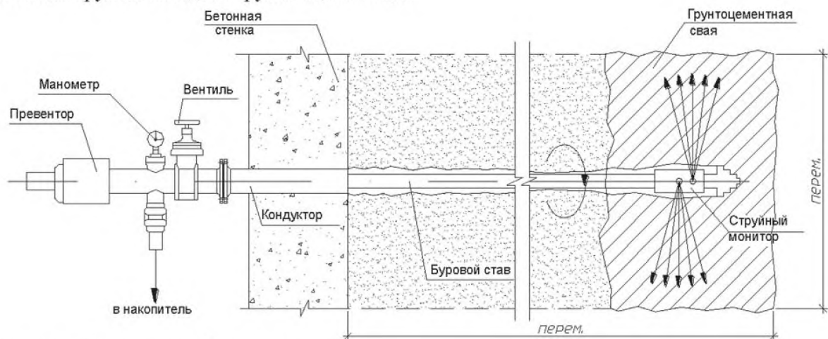
б) инъекция грунтов через буровой став
