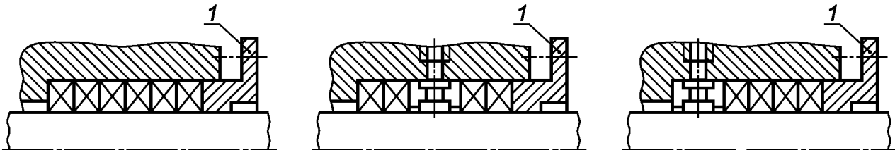
P1 — мягкий сальник (одинарная компоновка)**
