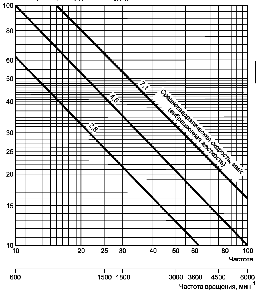
Рисунок Е.1 — Одиночная амплитуда A как функция частоты вращения для различных величин среднеквадратических скоростей
