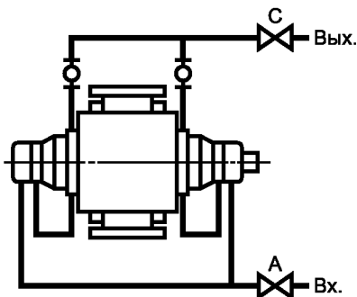
Схема Е Последовательное охлаждение камеры мягкого сальника и корпуса подшипника
