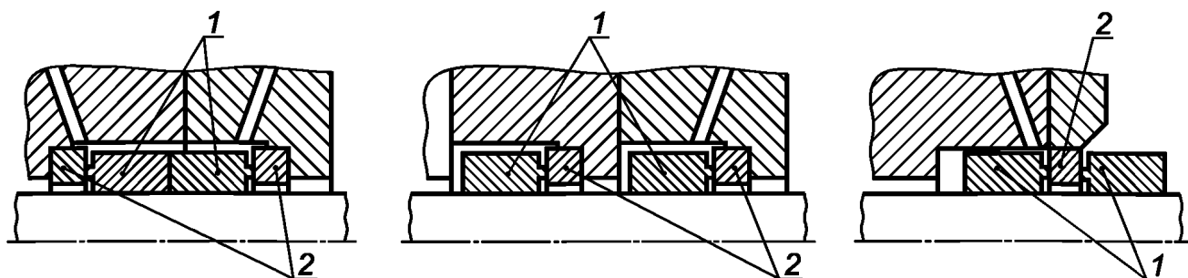
D1 — «спиной к спине»
