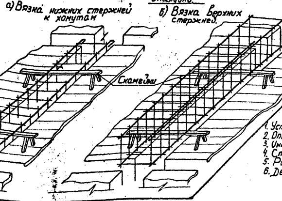
Схема вязки каркаса балки над коробом опалубки
