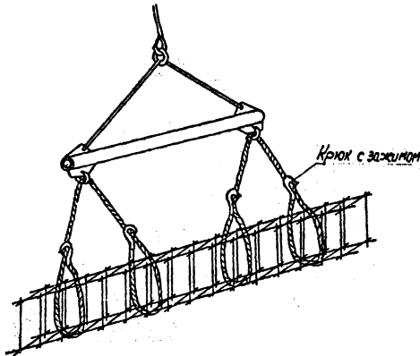
Схема строповки арматурного каркаса
