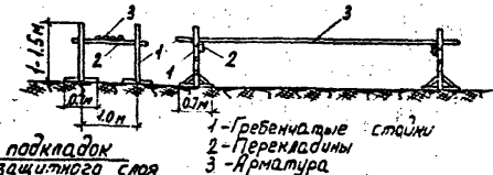
Деревянные стеллажи для арматуры
