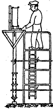
Схема сборки и вязки на днище короба с передвижных площадок и вышек.
