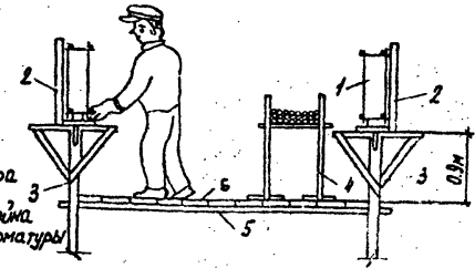
Деревянные стеллажи для арматуры
