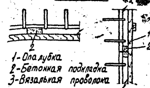
Установка подкладок для обеспечения защитного слоя бетона
