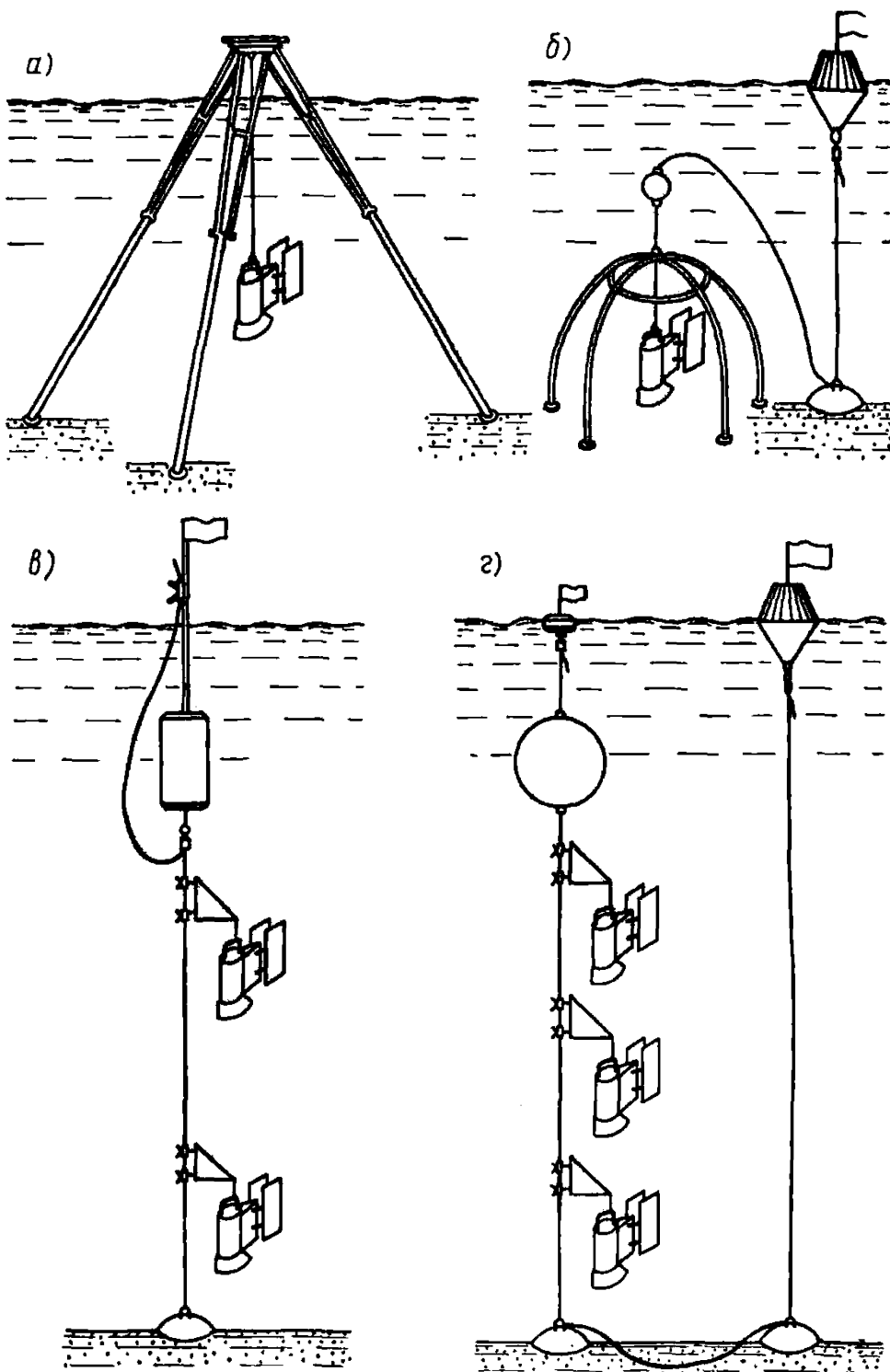
Рис. 77. Устройства для установки самописцев течений в водоемах a — на треноге; б — на каркасе типа «колокол»; в — на тросе с подтопленным несущим буюм; г — на тросе с подтопленным несущим и вынесенным сигнальным буюми
