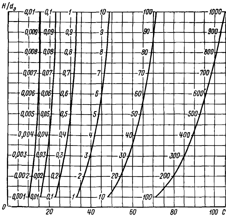
Рис. 35. Номограмма c = f\left(\frac{H}{d_3}\right)
