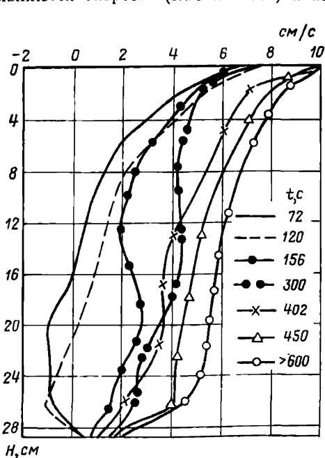
Рис. 62. Изменение по вертикали скорости развивающегося однонаправленного ветрового течения (данные эксперимента)
