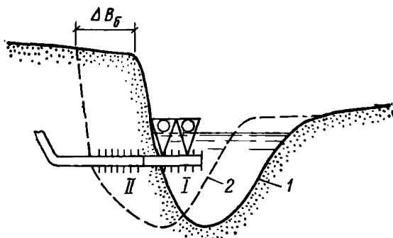
Рис. 11. Схема двухсекционного внутриводного выпуска на участке свободно меандрирующего русла
