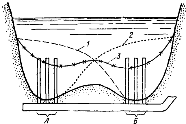
Рис. 5. Двухсекционный донный выпуск при побочном типе руслового процесса
