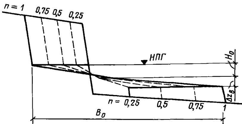
Рис. 32. Стадии развития береговой отмели
