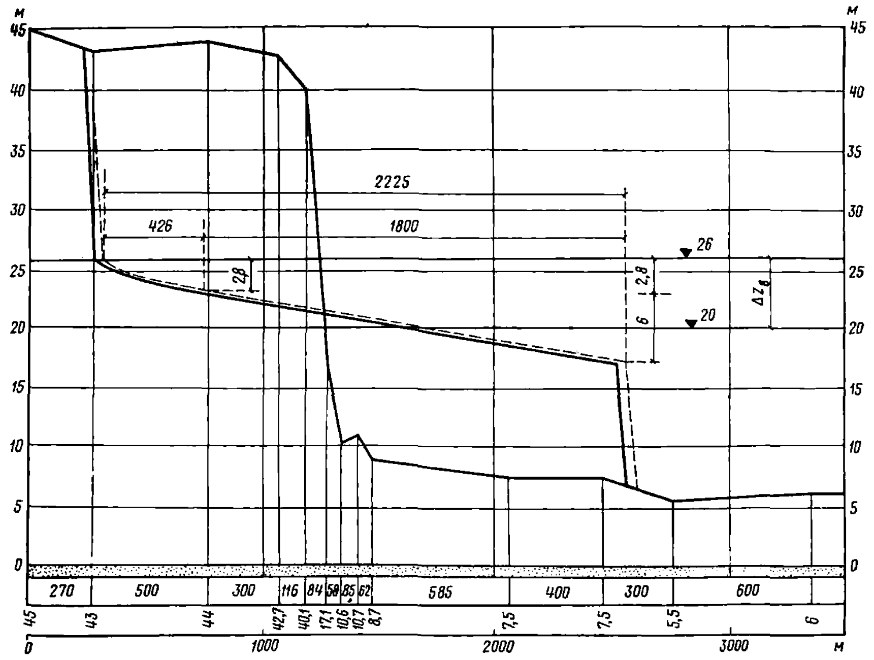
Рис. 85. Профиль береговых деформаций
