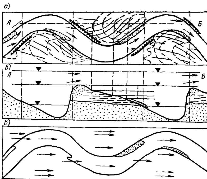
Рис. 56. Схема пойменного массива при ограниченном меандрировании
