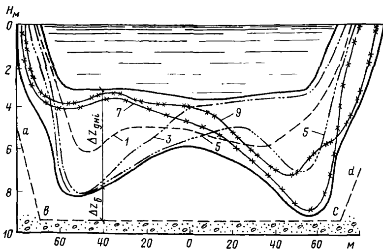
Рис. 1. Деформации русла при побочном режиме 1, 3, 5, 7, 9 — совмещенные поперечные профили; линия abcd — предельный запас к расчетному контуру размыва
