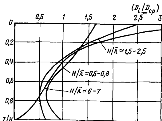
Рис. 14. Распределение безразмерных величин кинематического коэффициента турбулентной вязкости однонаправленного по глубине ветрового течения при различных значениях H_\lambda
