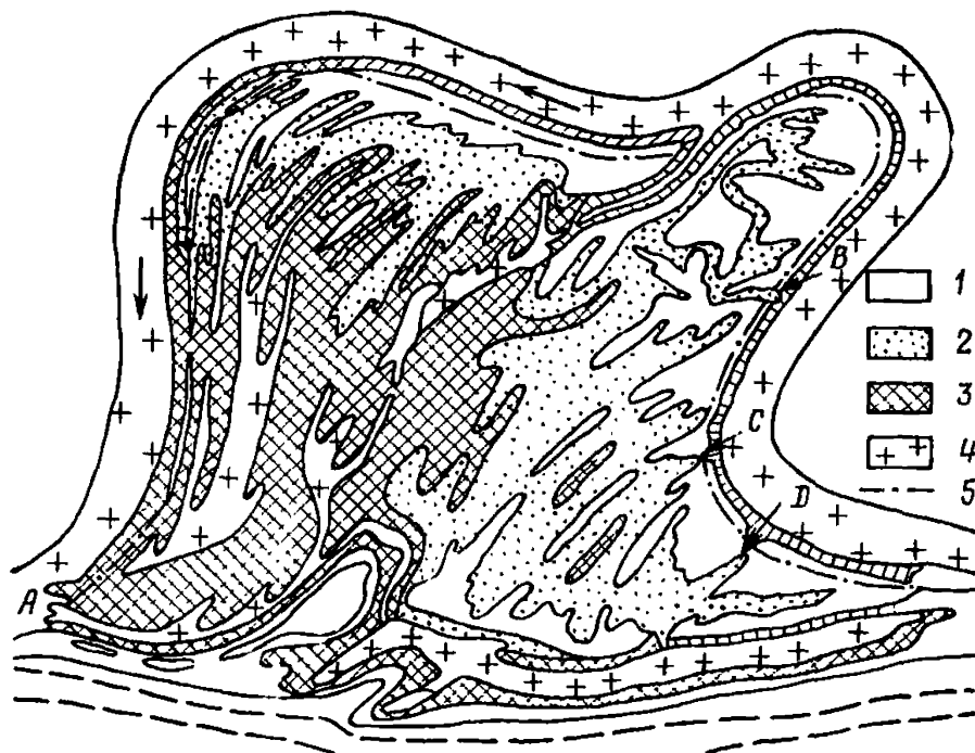
Рис. 51. пойменный массив при свободном меандрировании
