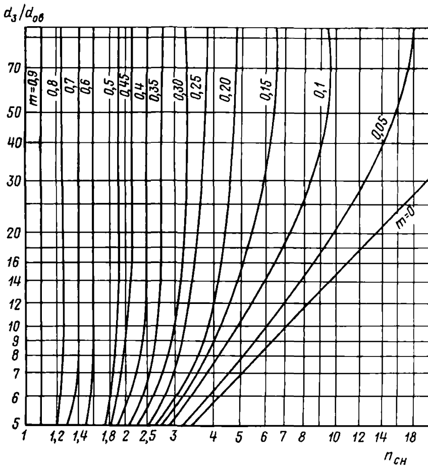
Рис. 38. Номограмма для определения начального разбавления в потоке
