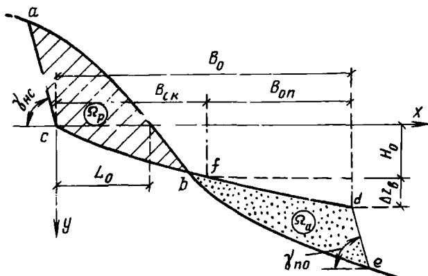
Рис. 27. Схема береговой отмели
