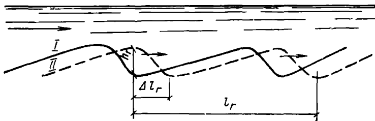
Рис. 55. Мелкие песчаные гряды
