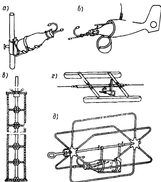
Рис. 80. Батометры различных типов для отбора проб воды на мутность
