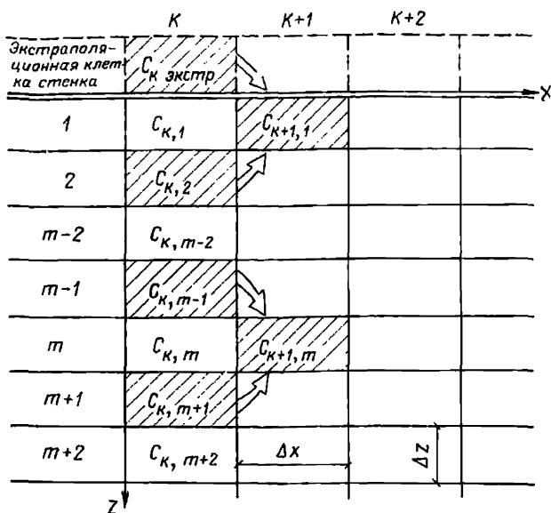
Рис. 41. Сетка к расчету турбулентной диффузии. Плоская задача
