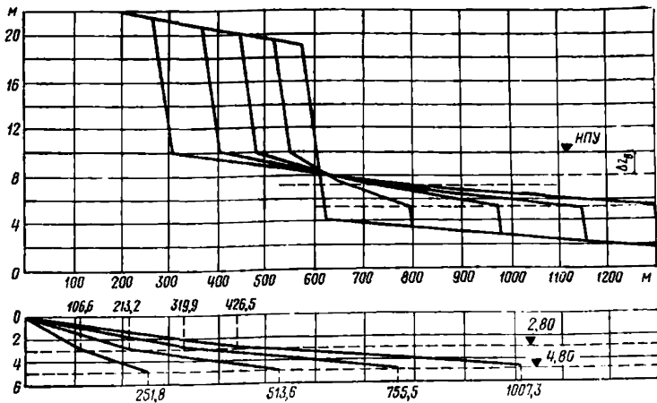
Рис. 86. Профиль прогноза береговых деформаций
