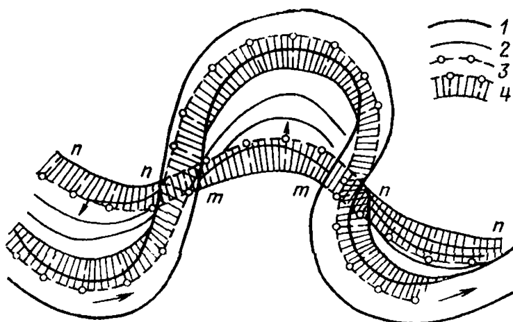
Рис. 60. Восстановление прежних положений русла по веерам перемещения
