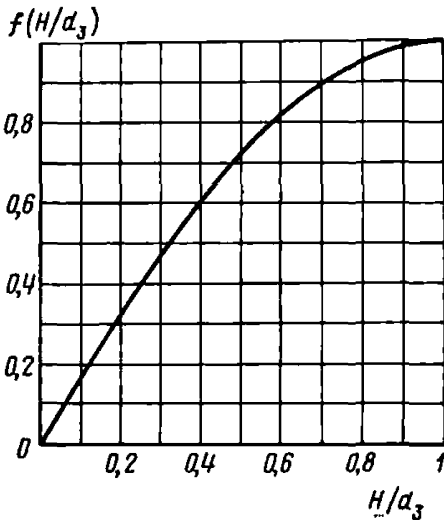
Рис. 38. Номограмма для определения начального разбавления в потоке
