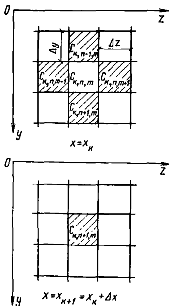
Рис. 40. Сетка к расчету турбулентной диффузии. Пространственная задача
