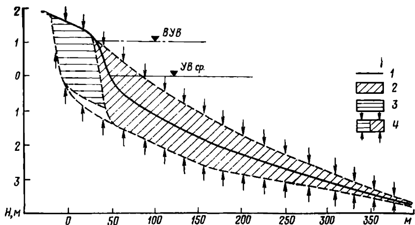
Рис. 25. Контуры высотных деформаций дна береговой отмели при длительном стоянии уровня на высоких отметках 1 — осредненный профиль; 2 — контуры призмы деформаций; 3 — контуры призмы дополнительных деформаций; 4 — результирующий контур высотных деформаций
