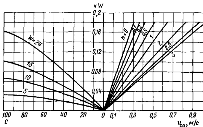
Рис. 36. Номограмма для определения средней скорости ветрового течения
