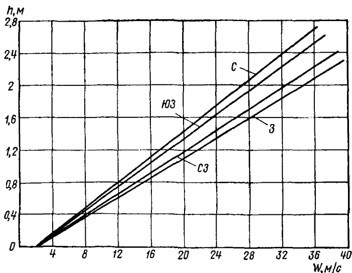
Рис. 82. График к расчету волнового режима водохранилища
