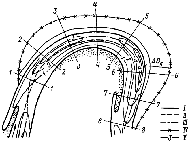
Рис. 2. Плановые деформации излучины при свободном меандрировании
