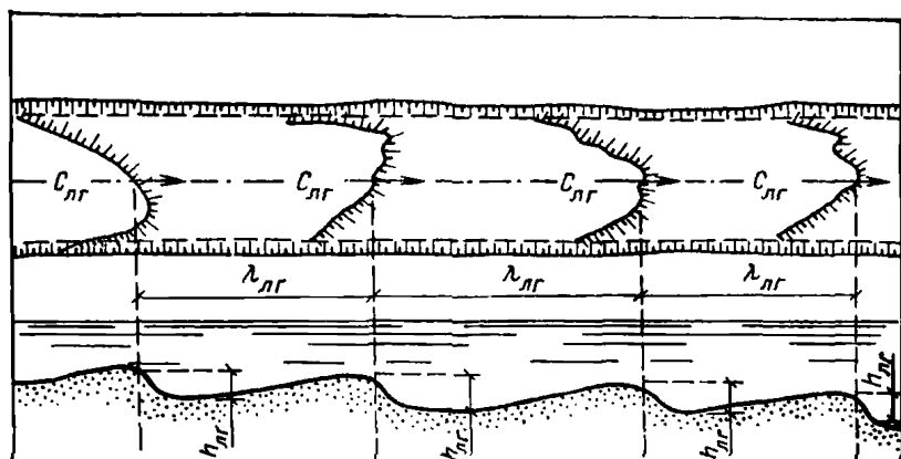
Рис. 47. Ленточногрядовый тип руслового процесса
