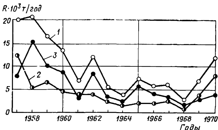
Рис. 21. Изменение по годам вдольбереговых перемещений наносов 1 — суммарное; 2 — вправо; 3 — влево от створа
