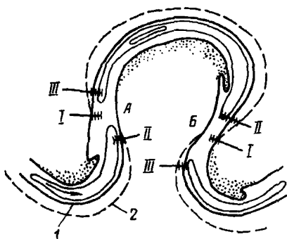
Рис. 9. Расположение створов выпусков на свободно меандрирующей излучине А — верхний перекаат; Б — нижний перекаат; I — створ на перекаате, II — створ в конечном участке плеса; III — створ в начальном участке плеса; 1 — начальное положение берега; 2 — конечное положение берега
