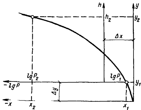
Рис. 83. График к расчету волнового режима водохранилища
