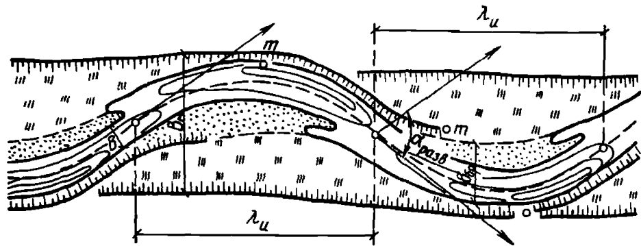
Рис. 48. Побочный тип руслового процесса
