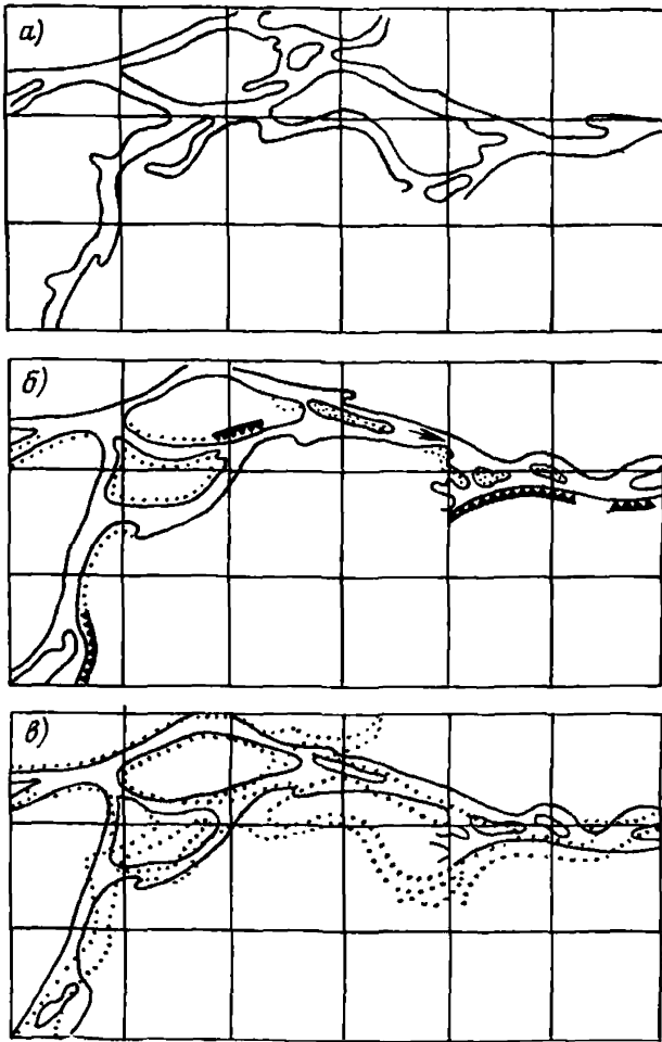
Рис. 59. План участка реки а — по съемке 1913 г.; б — по съемке 1960 г.; в — совмещенные планы 1913 и 1960 гг.
