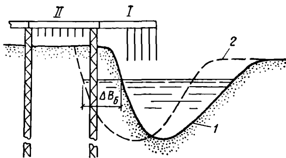
Рис. 10. Схема двухсекционного надводного выпуска на участке свободного меандрирования русла
