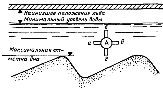
Рис. 4. Размещение внутриводного выпуска при ленточногрядовом типе руслового процесса
