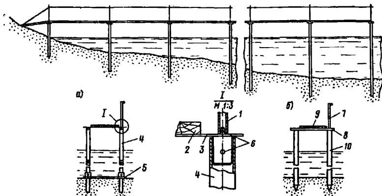
Рис. 78 Эстакада
