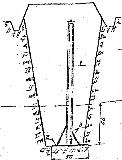
Грунтавый репер для труднопроходимых районов
