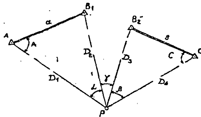
Рис 3.1 Схема определения места на галсе двумя секстанами а) по смежным пунктам б) по двум парам пунктов.
