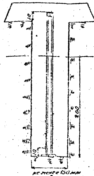
Грунтавый репер для районов вечной мерзлоты
