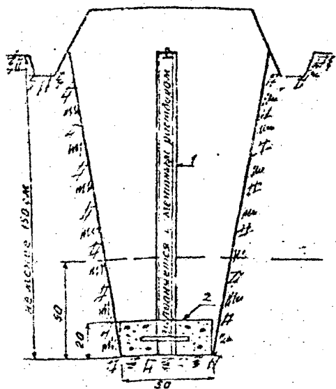
Грунтавый репер
