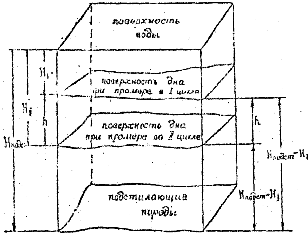
Рис. 5.1 Схема участка горных работ от поверхности воды до подстилкающих пород и поверхностей дна.
