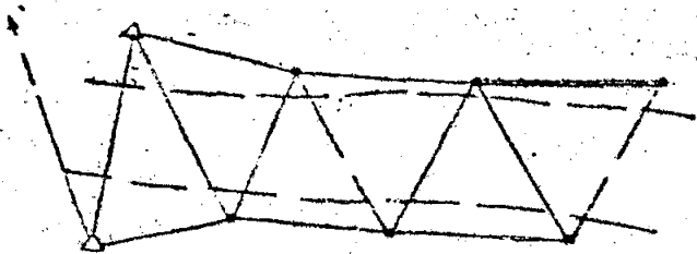
Цепочка треугольников
