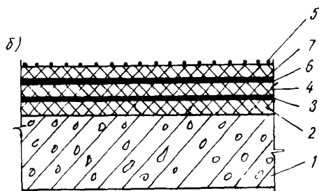
Рис. I. Рекомендуемые типы однослойной (а) и двухслойной (б) оклеечной гидроизоляции 1 - плита перекрытия; 2, 4, 7 - слой клея; 3, 6 - полиэтиленовая пленка; 5 - посыпка кварцевым песком
