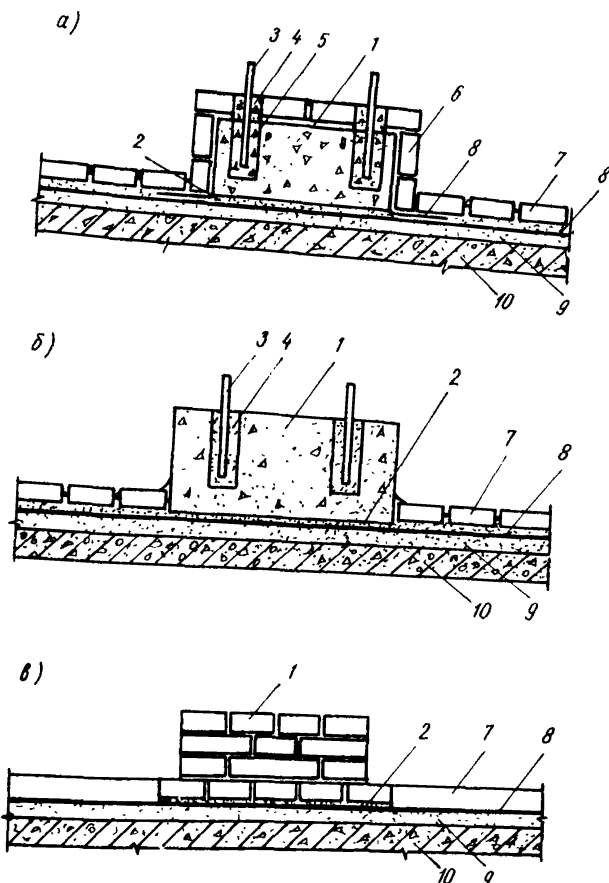
Рис. 2. Рекомендуемые конструкции фундаментов под оборудование
