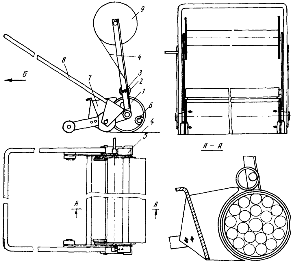
Рис. 5. Устройство для оклеивания полиэтиленовой пленкой
