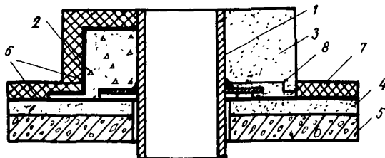
Рис. 3. Схема пропуска коммуникаций через покрытия
