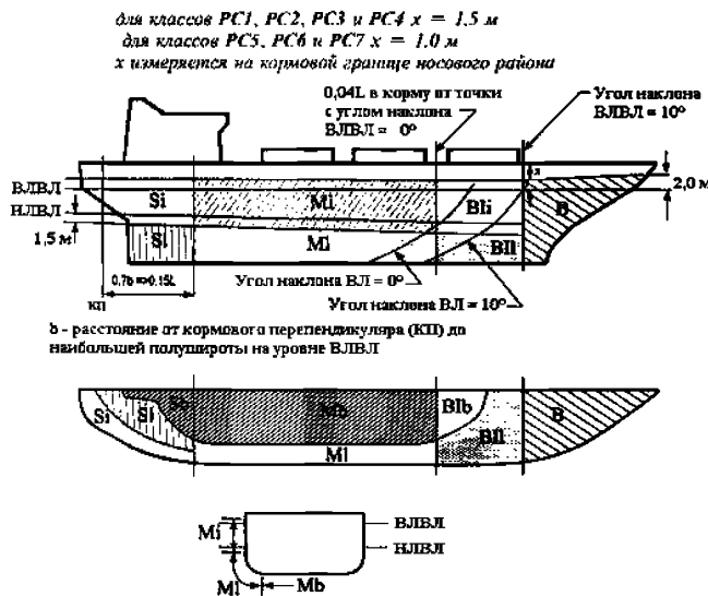
Рис. 1.2.2.1 Границы районов корпуса судна
