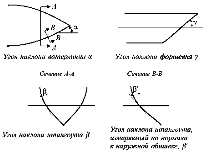
Рис. 1.2.3.2.1.1.1 Определение углов наклона
