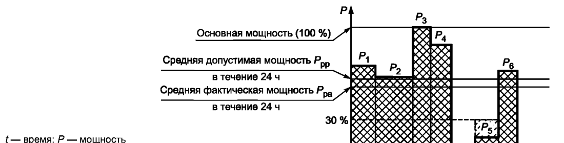
Рисунок 2 — График-иллюстрация основной мощности (PRP)
