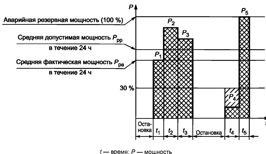
Рисунок 4 — График-иллюстрация аварийной резервной мощности (ESP)
