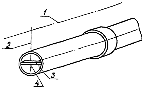
Рис.9. Схема центровки труб со стороны торца
