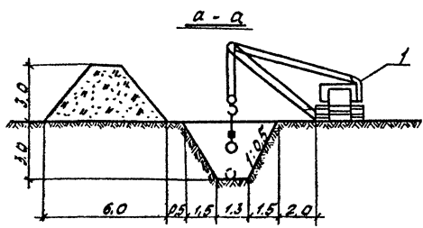
Рис. 1 Схема производства работ
