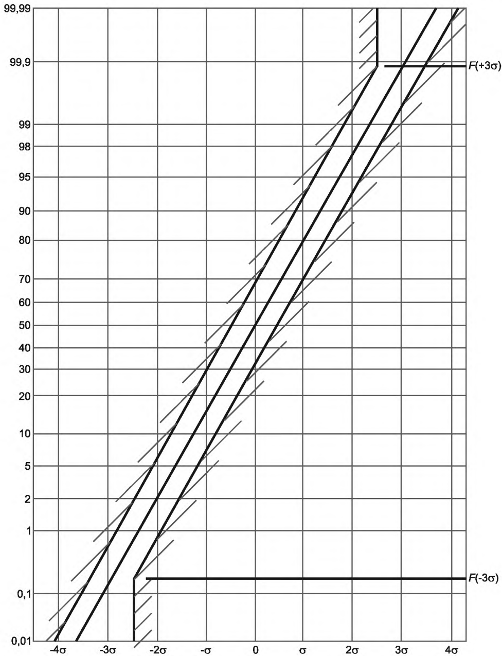
Рисунок 5 — Поля допуска для интегральной плотности распределения вероятности
