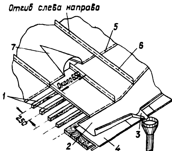
Конструкция кровли
