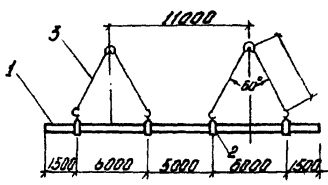
Рис.4. Схема строповки звена труб. 1 - звено трубы ( \varnothing=20m ) 2 - П-820 ÷ П-1020 3 - строп 2х ветвевой
