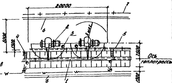
Рис.3. План укладки стальных труб в траншею 1 - траншея с подготовленным основанием; 2 - кран КС-2561 (2шт); 3 - рабочие места такелажников; 4 - лестница (2шт); 5 - складирование труб; 6 - лифтовые канаты; 7 - граница охранной зоны. 8 - передвижная электростанция.
