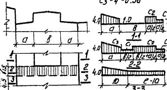
Схема снеговых нагрузок на покрытие у торца фонаря в месте перелома высот между пролетами одного направления
