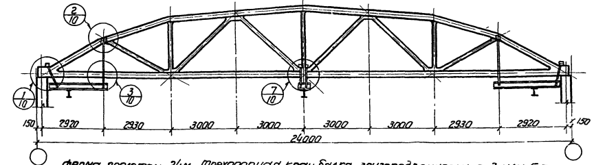
Ферма пролетом 24 м. трехпарная кран-балка грузоподъемностью 3 т. 5 т.
