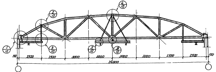
Ферма пролетом 24 м. 2 кран-балки грузоподъемностью 2 т. 3 т. с переходным мостиком.
