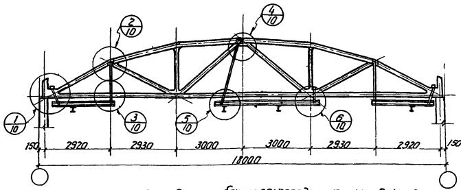
Ферма пролетом 18 м. 2 кран-балки грузоподъемностью 2 т. 3 т. с переходным мостиком.
