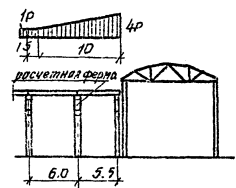
Схема снеговых нагрузок на покрытие в месте перелома высот при взаимно перпендикулярных направлениях
