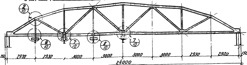
Ферма пролетом 24 м. Манарельсы (4 груза по 3,9 т.)
