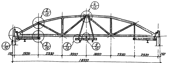
Ферма пролетом 18 м. 2 кран-балки грузоподъемностью 2 т. 3 т.
