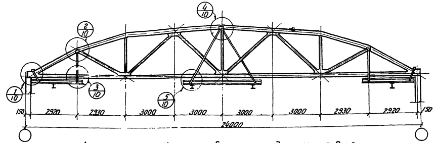
Ферма пролетом 24 м. 2 кран-балки грузоподъемностью 2 т. 3 т.
