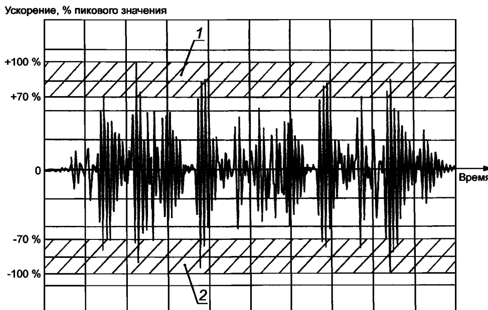
Рисунок 1 — Пример отклика осциллятора на заданный временной сигнал возбуждения
