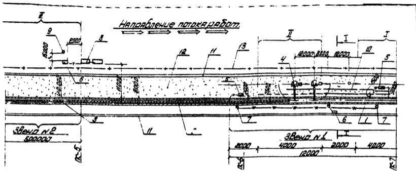
Рис. 1. Строительный план
