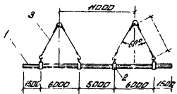
Рис. 4. Схема строповки звена тр. б. 1- звено трубы ( e=20m ); 2- \Gamma-325/4шт ; 3- строп 2х ветвями Q=4,0 тс
