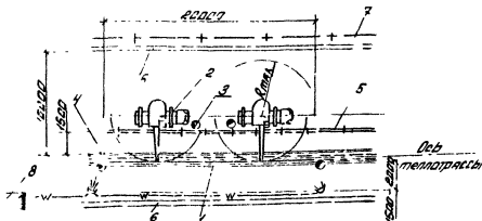
Рис. 3. План укладки стальных труб в траншею 1- траншея сложенная минимальными лотками; 2- края КС-256 (2 шт); 3- рабочие места тампаляж- ников; 4- лестницы (2 шт); 5- скрепление труб, 6- ливневые канавы; 7- граница охранной зоны 8- переувлажненная электростанция.
