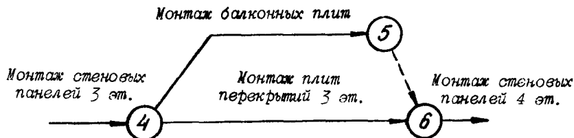
Рис.2. Изображение параллельных работ.
