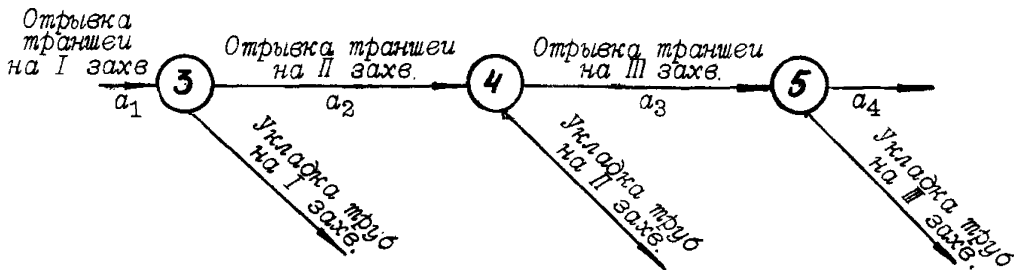
Рис. 3. Разбивка работы на части при осуществлении потока
