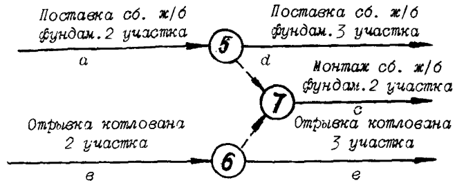
Рис. 5. Изображение зависимостей между работами.
