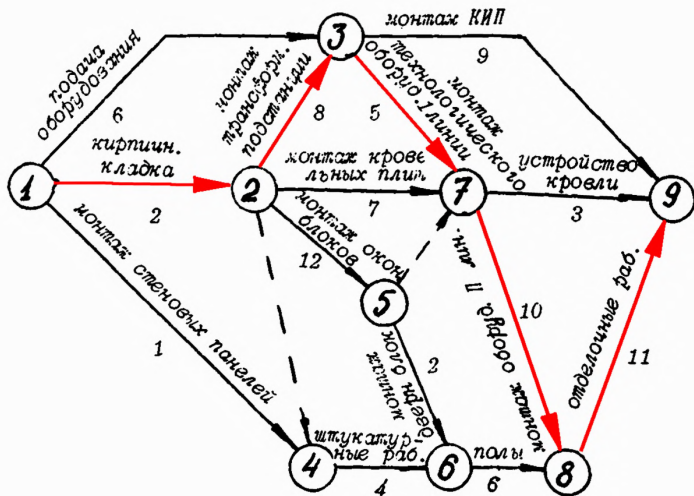
Рис.10. Сетевой график.
