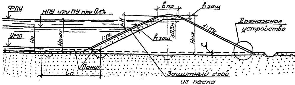
Черт. 42 Поперечные профили плотин из глинистых грунтов H_{пл} \leq 15м ; H_n \leq 13м .
