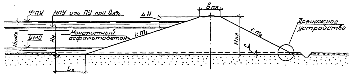
Черт. 4.7 Поперечные профили плотин из песка (за исключением пылеватого и мелкого, при \gamma_f > 30^\circ ) с экраном из асфальтобетона H_{пл} \leq 15 м; H_n \leq 13 м. Коэффициенты откосов принимаются по табл. 4.5.
