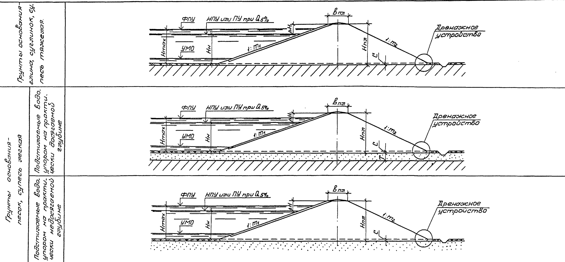
Черт. 43. Поперечные профили плотин из песка средней крупности или мелкого H_{пл} \leq 15 м ; H_{пл} \leq 13 м . Коэффициенты откосов (при \varphi \geq 30^\circ ) принимаются по таблице 43.
