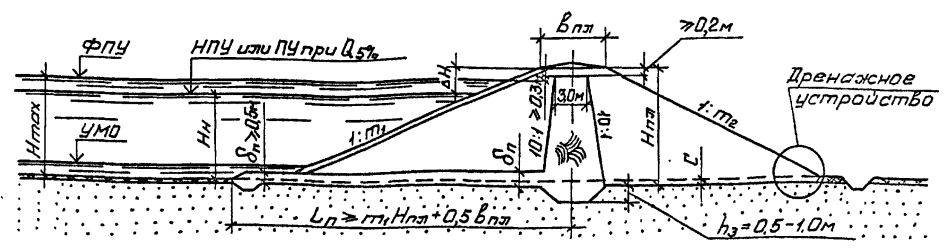
Черт. 4.4. Поперечные профили плотин из песка (за исключением пылеватого) с ядром из глинистых грунтов H_{пл} \le 15м ; H_N \le 13м .
