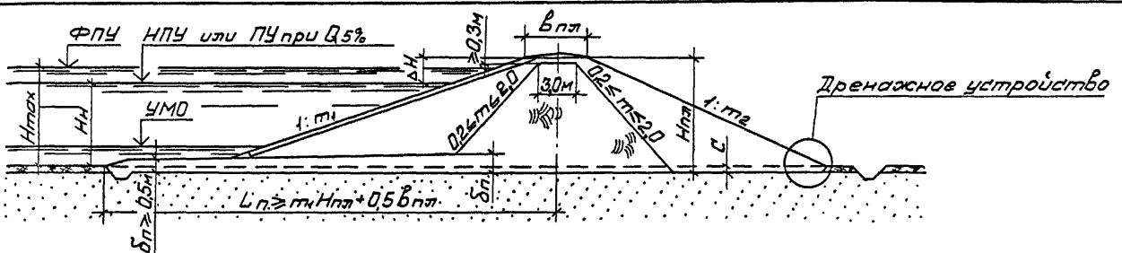
Черт. 48 Поперечные профили плотин из двух или трех видов грунта; H_{пл} \leq 15м ; H_{н} \leq 13м . Коэффициенты откосов m_1 и m_2 принимаются в зависимости от грунта, слагающего откос: при глинистых грунтах - по табл. 42, при песчаных грунтах - по табл. 44.
