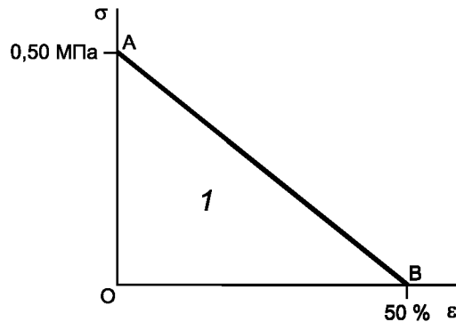
Рисунок 1 — Треугольник зависимости напряжений от деформации
