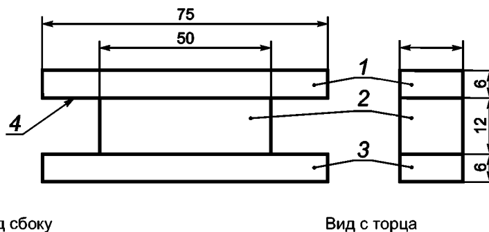
1 — стекло; 2 — герметик 3 — стекло; 4 — поверхность стекла, которая может быть с покрытием
