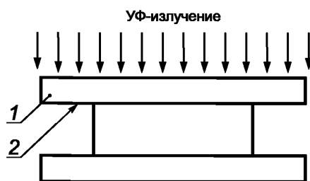
1 — стекло; 2 — испытываемая поверхность (может иметь покрытие)
