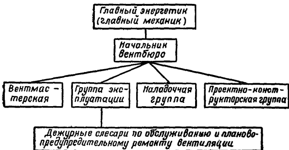
Рис. 1 Структурная схема вентбюро типа А
