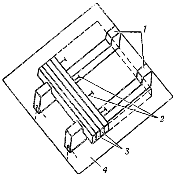
Рис. 36. Приспособление для сплачивания дверного полотна:
