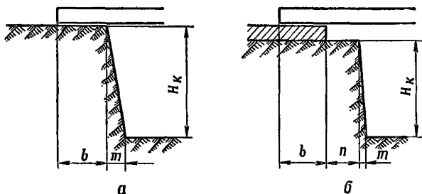
Рис. 11. Схемы опирания покрытия: а — на берму котлована; б — на опорную площадку с оставлением ненагруженной бермы
