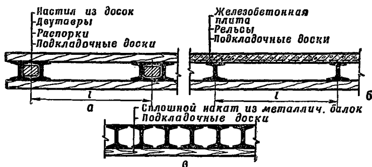
Рис. 34. Варианты конструкции покрытий с применением металлических балок:
