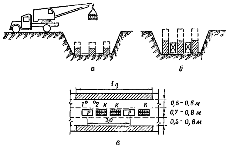
Рис. 12. Схема производства работ при кладке кирпичных стен: a — кладка первого яруса; б — кладка второго яруса; в — схема организации рабочего места на делянке; 1, 2 — звено каменщиков; P — раствор; K — кирпич; l_d — длина делянки
