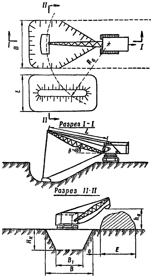
Рис. 8. Схема производства работ по отрывке котлована экскаватором, оборудованным драглайном, при торцевой проходке: e = 1 \text{ м}
