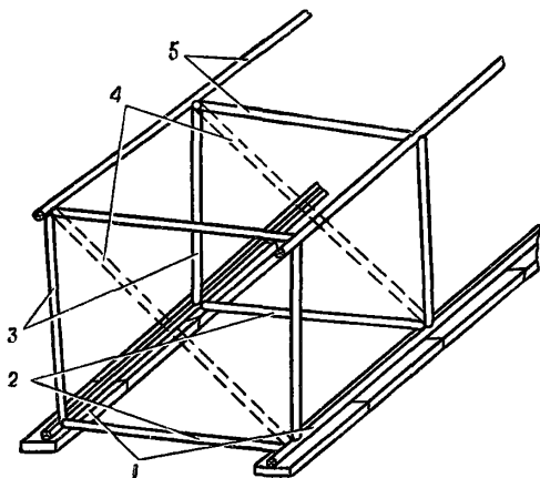
Рис. 24. Схема устройства каркаса из круглого леса:
