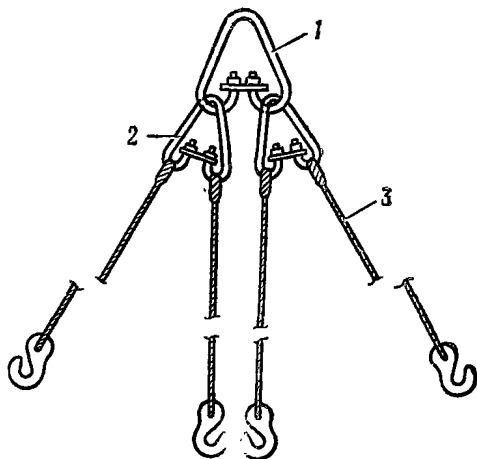
Рис. 14. Траверса «паук» для монтажа крупных бетонных блоков:
