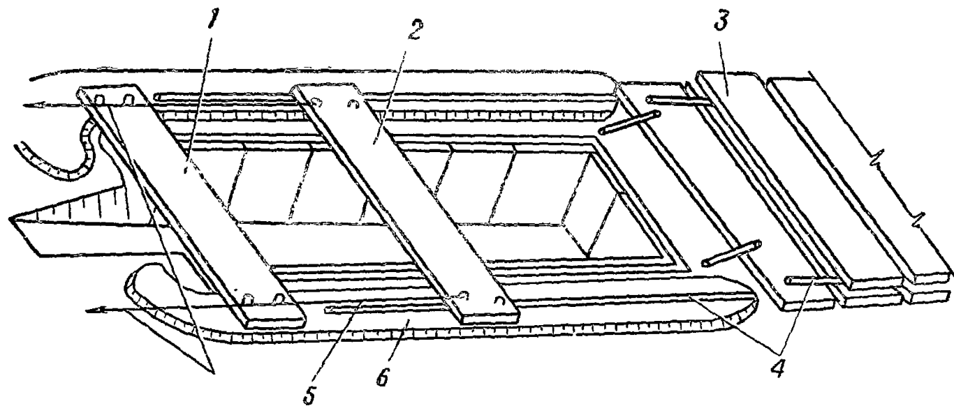
Рис. 33. Схема укладки плит покрытия вручную способом надвигки: 1 — плита в проектном положении; 2 — надвигаемая плита; 3 — штабель плит (2 плиты по высоте); 4 — лежни из подтоварника \Phi 10–12 см; 5 — тросы (канаты) для перемещения плит; 6 — грунтовая подсыпка толщиной 10–12 см
