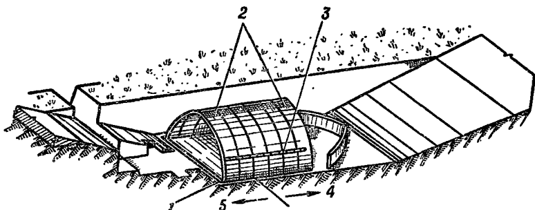
Рис. 29. Сборка остова сооружения из элементов комплекта «Арка»:
