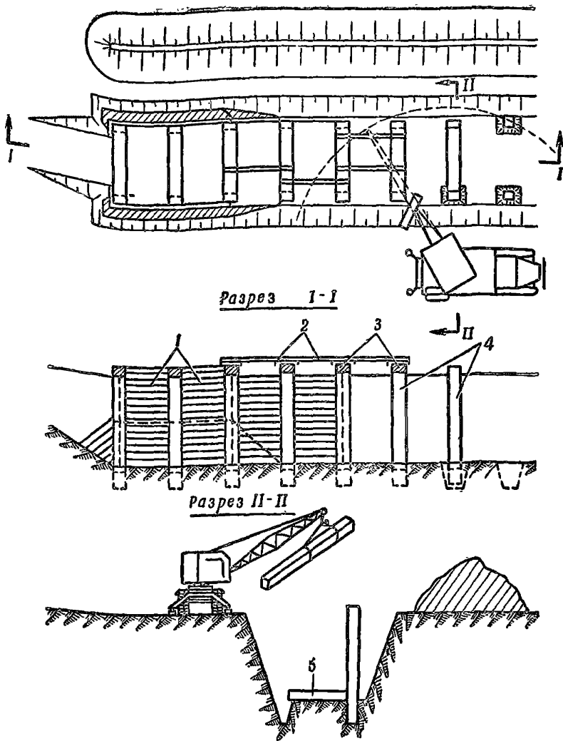
Рис. 25. Схема производства работ по возведению остова из железобетонных рам с забиркой стен из дощатых щитов: 1 — дощатые щиты; 2 — струбцины для временного крепления рам; 3 — ригели; 4 — стойки; 5 — нижние распорные элементы
