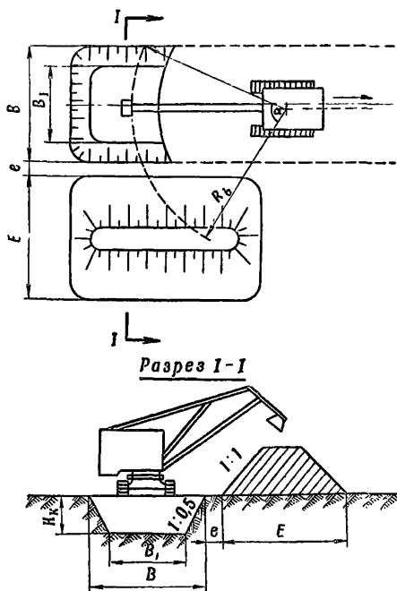
Рис. 6. Схема производства работ по отрывке котлована экскаватором с обратной лопатой при торцовой проходке: e = 1 \text{ м} , \alpha = 90-100^\circ
