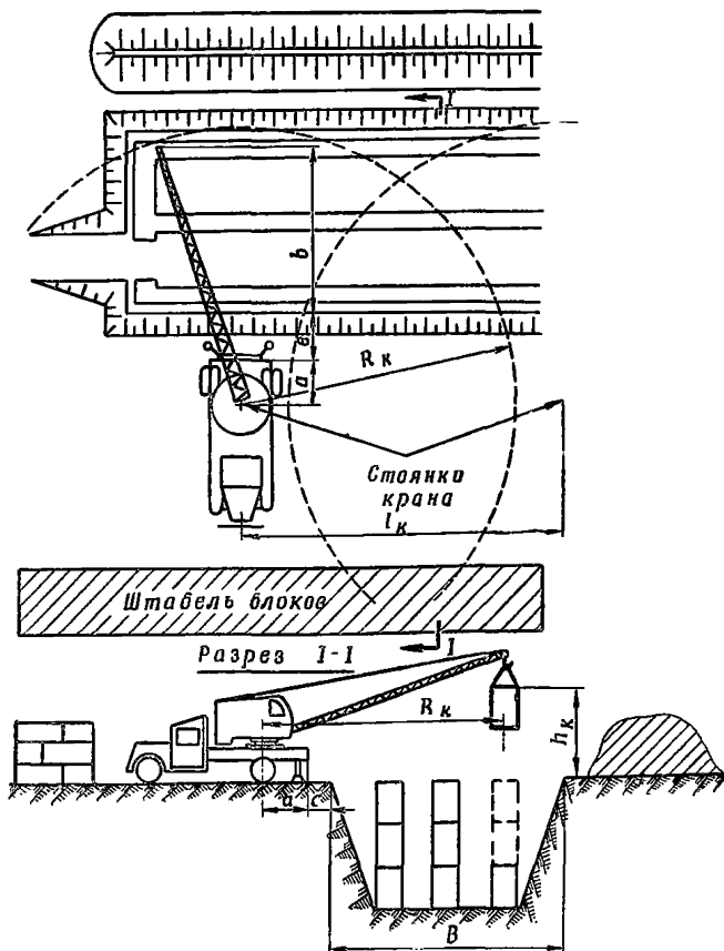
Рис. 13. Схема производства работ по монтажу стен из крупных бетонных блоков с помощью автокрана:
