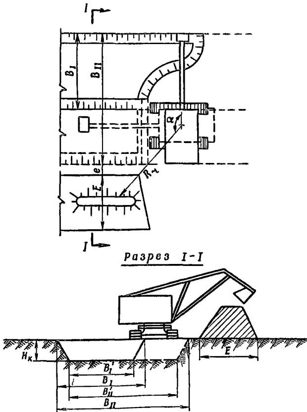
Рис. 7. Схема производства работ по отрывке котлована экскаватором с обратной лопатой при боковой (контур котлована показан сплошными линиями) и комбинированной (пунктирными линиями) проходках:
