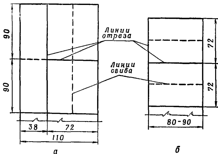
Рис. 15. Схема раскроя ткани для пошивки грунтонабивных мешков:
