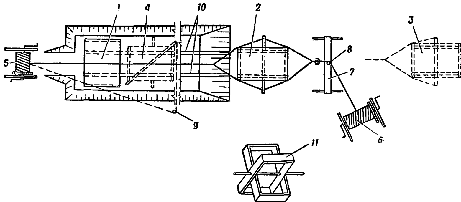
Рис. 31. Схема производства работ по укладке звеньев труб в котловане с помощью двух ручных лебедок:
