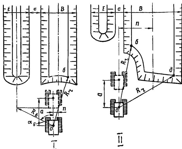
Рис. 9. Разбивочные схемы котлованов:
