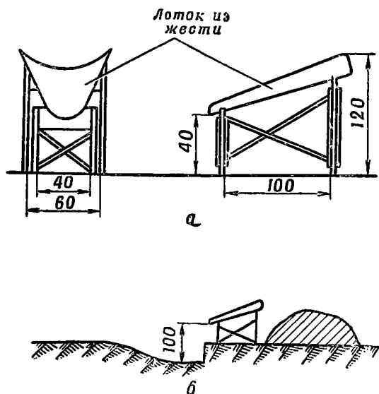
Рис. 16. Переносный лоток для заполнения мешков грунтом:
