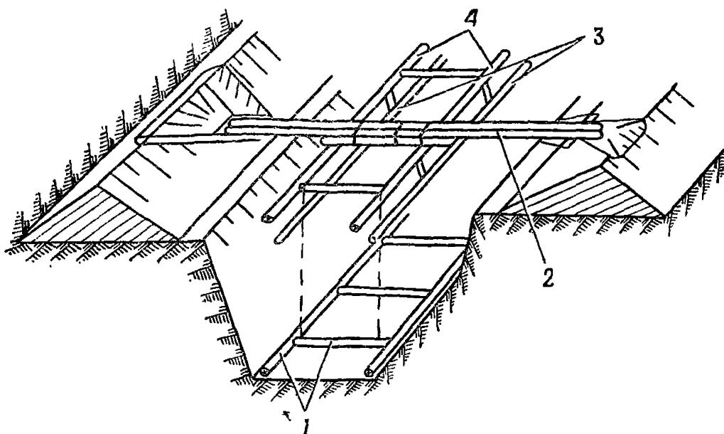
Рис. 22. Схема укладки нижних и верхних опорных рам: 1 — нижняя опорная рама; 2 — удлиненные элементы наката; 3 — монтажные жерди; 4 — верхняя опорная рама
