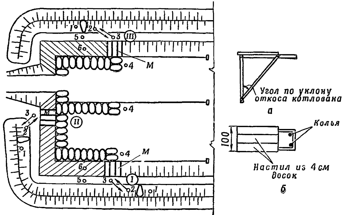
Рис. 17. Примерная схема организации работ при возведении стен из грунтонабивных мешков тремя звеньями:
