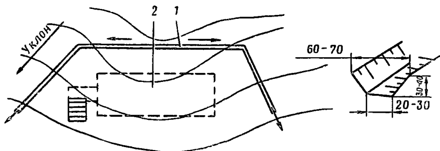
Рис. 4. Схема поверхностного водоотвода при расположении сооружения на косогоре: 1 — водоотводная канава; 2 — сооружение
