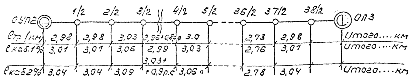
Схема размещения НУП
