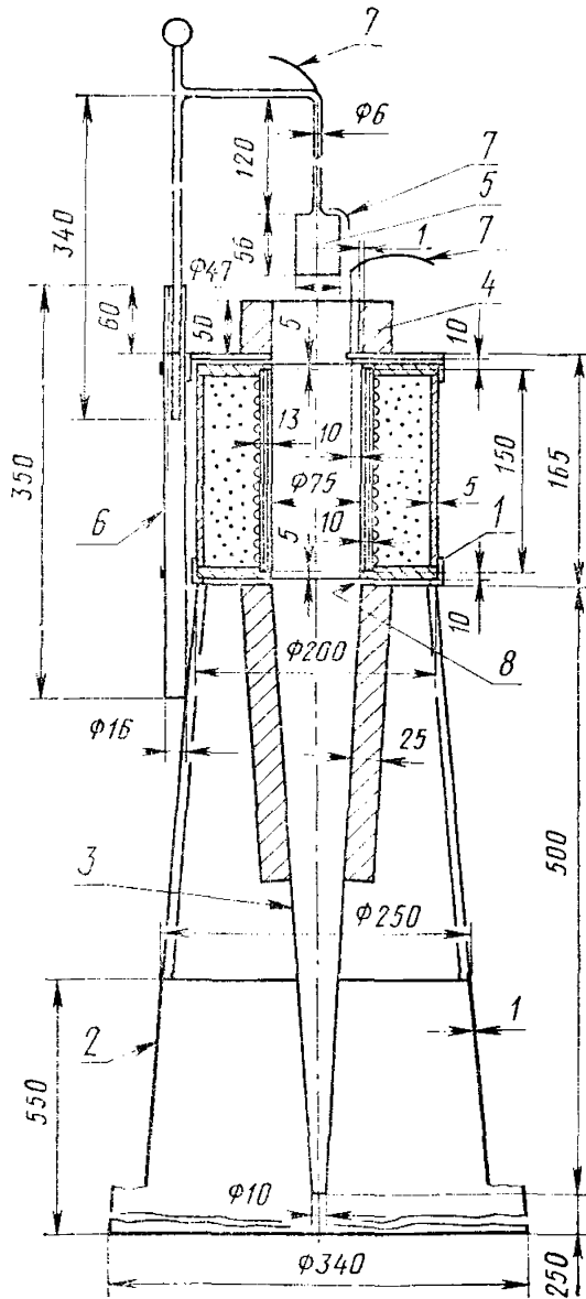
1—печь; 2—опорная станина; 3—стабилизатор; 4—защитный экран; 5—держатель образца; 6—направляющая планка; 7—термопара; 8—асбестовая прокладка.
