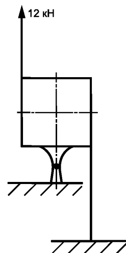
Рисунок 2 — Подвижное устройство
