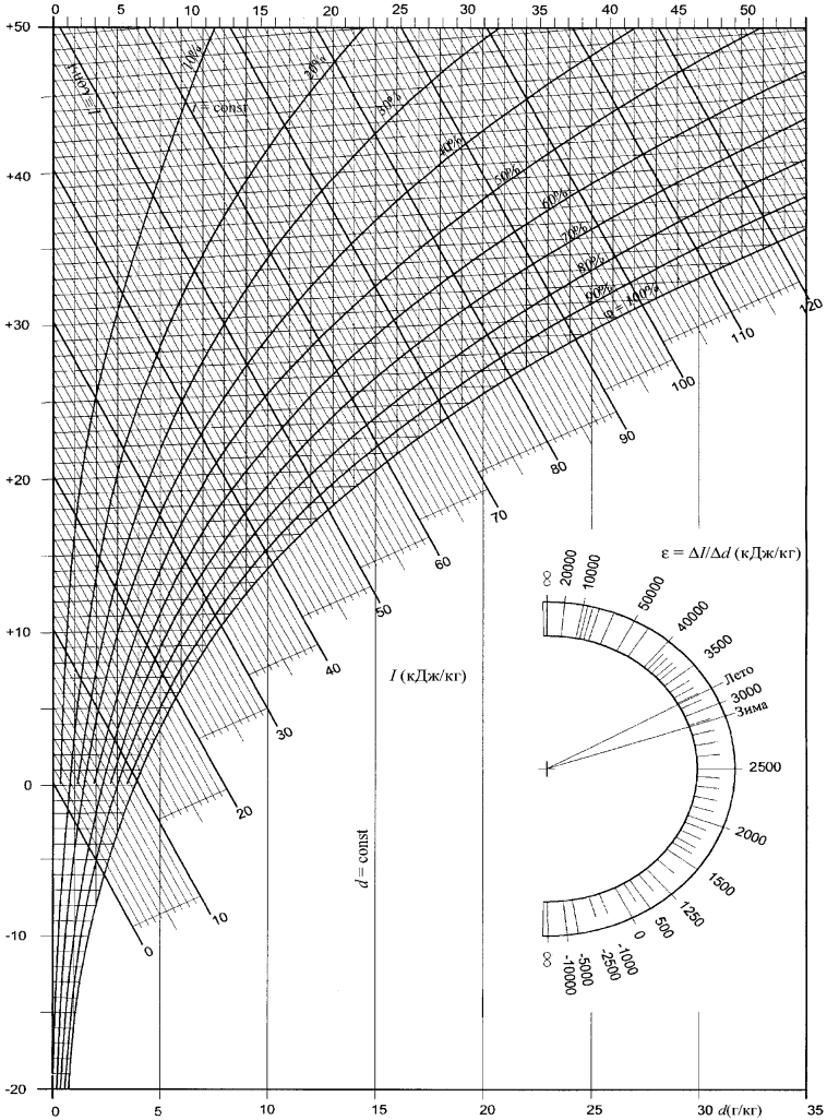
J - d диаграмма влажного воздуха
