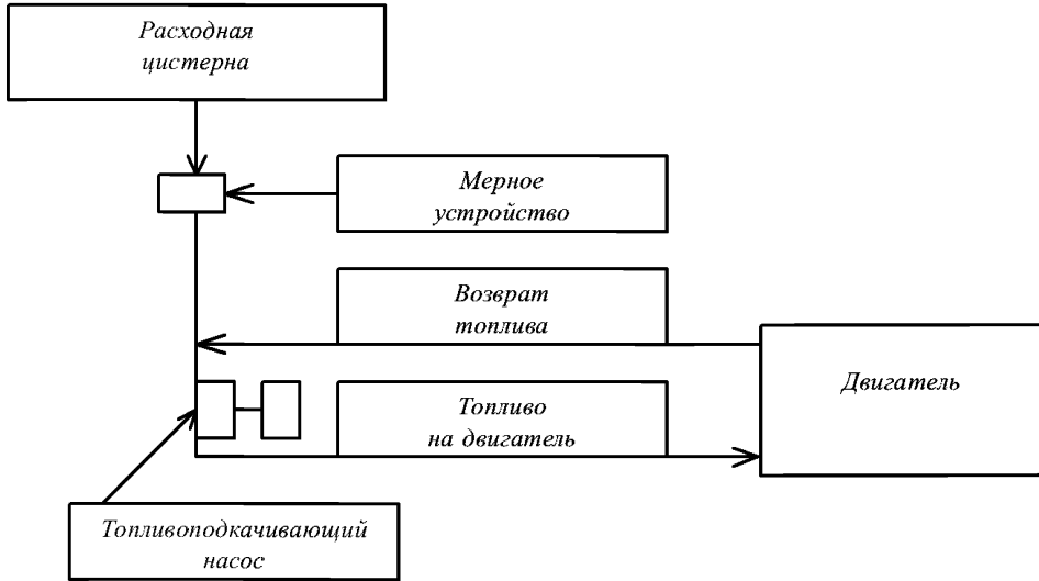
Рис. 4.1 Упрощенная схема топливоподающей системы
