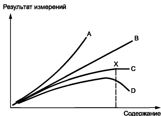
Рисунок 1 — Зависимость результата измерения от содержания загрязняющего вещества
