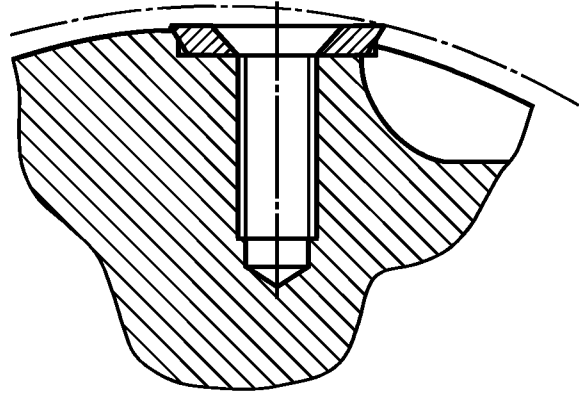
Крепление прижимным винтом со стороны задней поверхности режущей пластины
