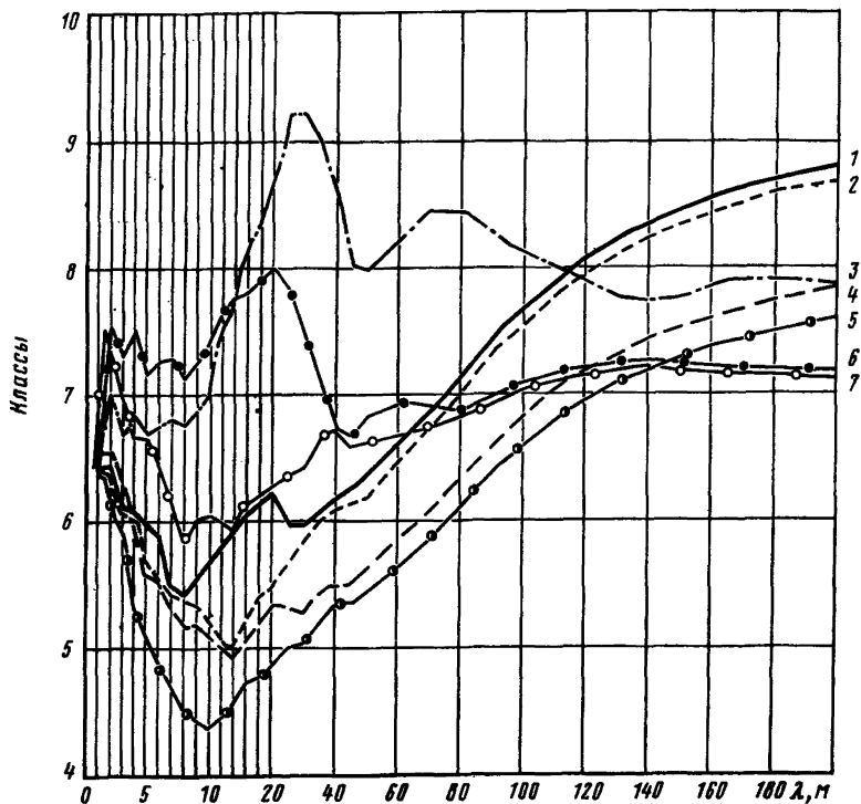
Рис. 1. Огибающие классов обращающегося подвижного состава:
