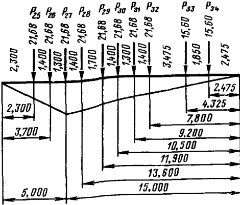
Рис. П.1.13. Линия влияния усилия при \lambda=20 м, \alpha=0,25
