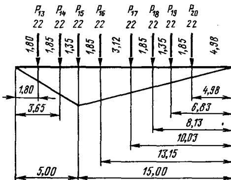
Рис. П.1.6. Линия влияния усилия при \lambda=20 м, \alpha=0,25
