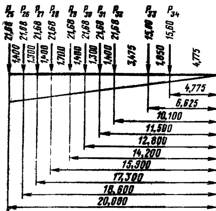
Рис. П.1.12. Линия влияния усилия при \lambda=20 м, \alpha=0,0
