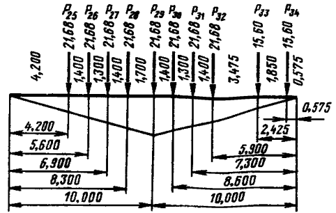
Рис. П.1.14. Линия влияния усилия при \lambda=20 м, \alpha=0,5
