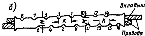
а — зажим для алюминиевых и стальных проводов; б — зажим для сталеалюминиевых проводов
