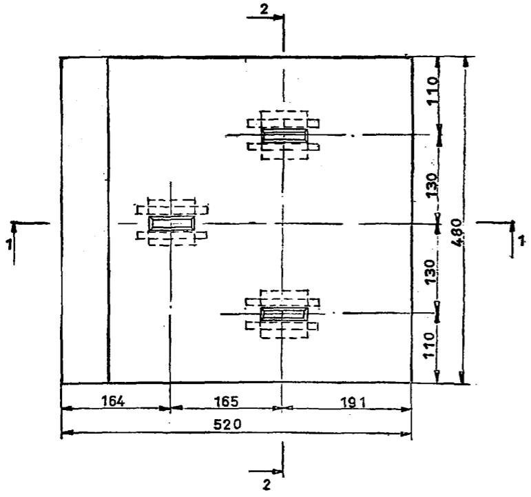
ПЛАН
