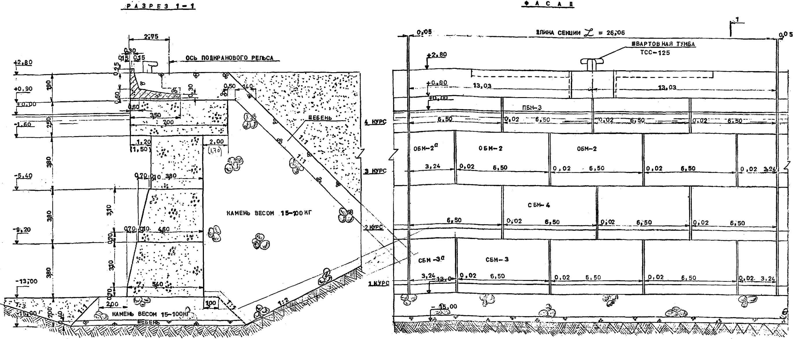
ОБЪЕМЫ РАБОТ НА 100 ПОГ. МЕТРОВ
