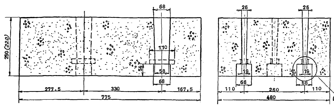
РАЗРЕЗ 1-1
