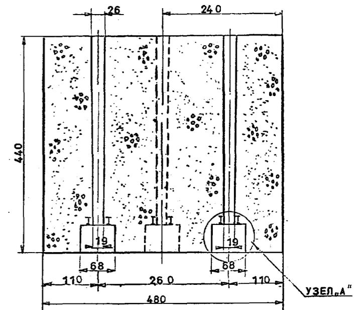
РАЗРЕЗ 2-2
