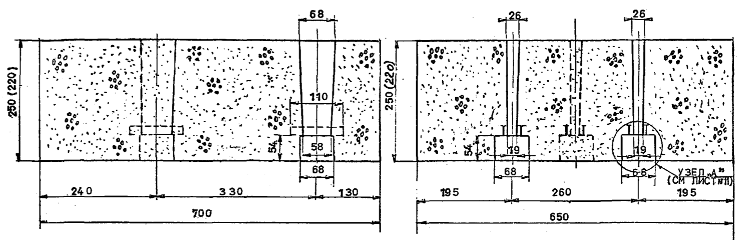
РАЗРЕЗ 1-1
