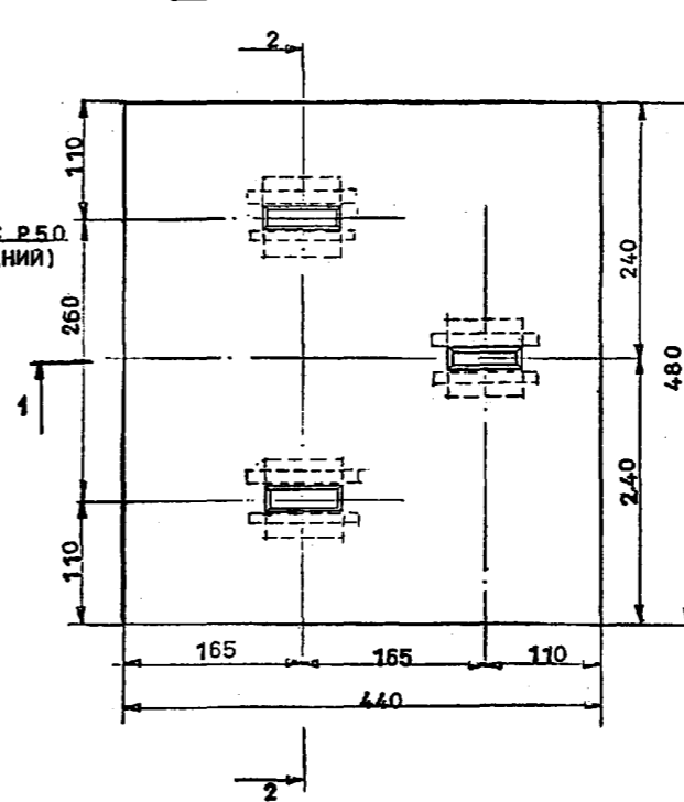
ПЛАН
