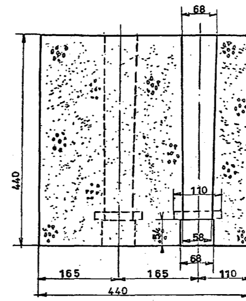
РАЗРЕЗ 1-1
