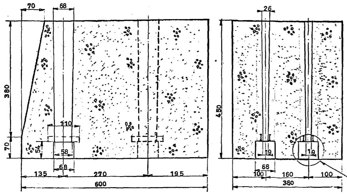
РАЗРЕЗ 1-1
