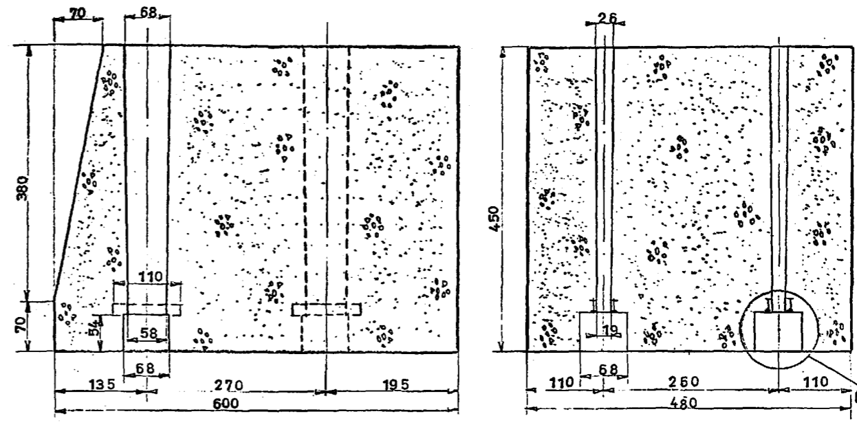
РАЗРЕЗ 1-1
