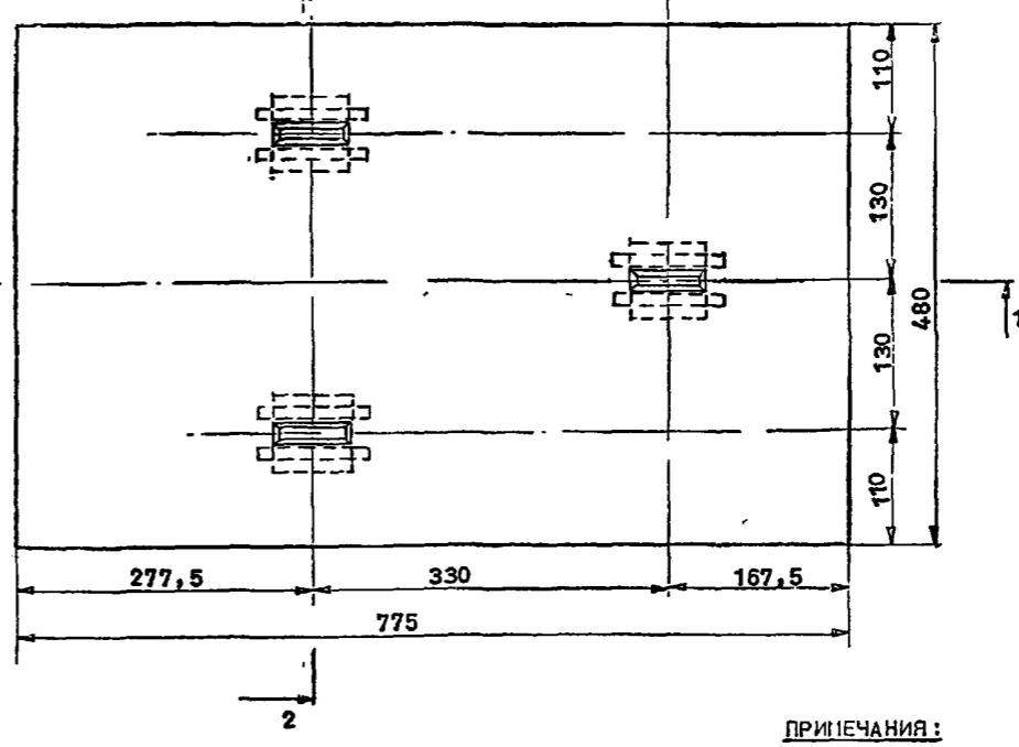
ПЛАН
