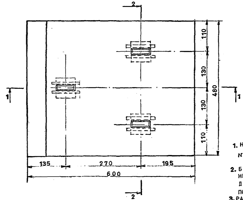
ПЛАН
