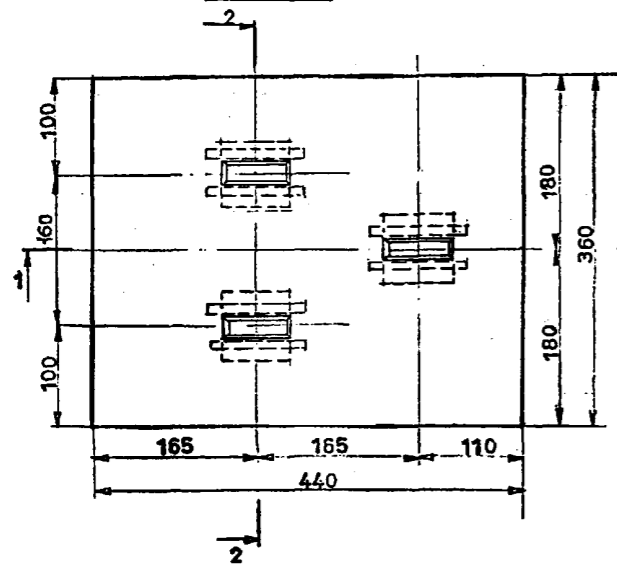
ПЛАН
