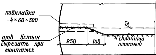
Деталь монтажного стыка днища
