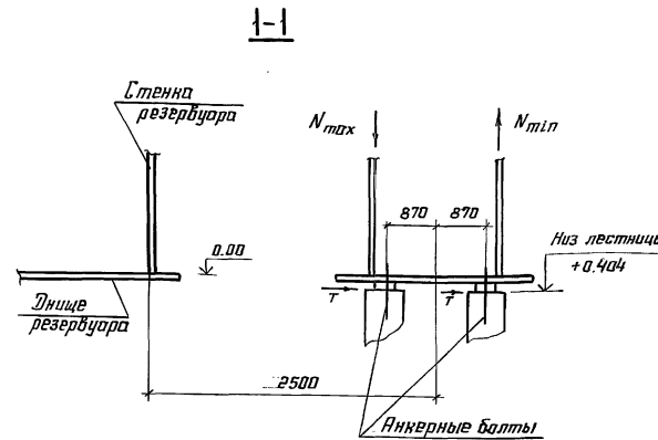
Анкерный болт
