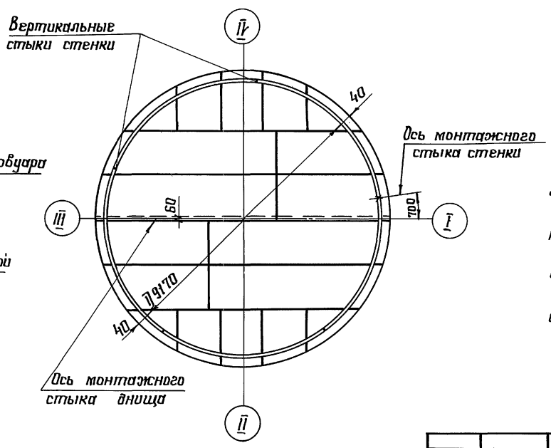
План днища
