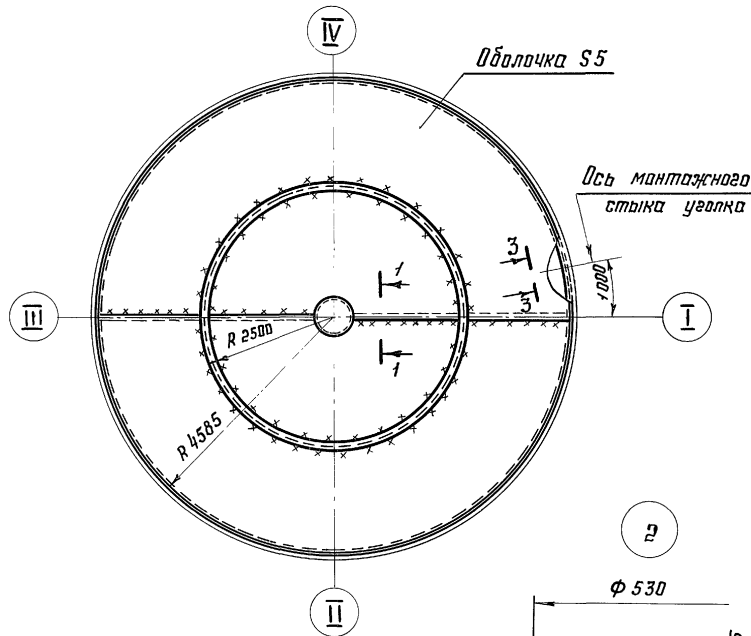
План крыши
