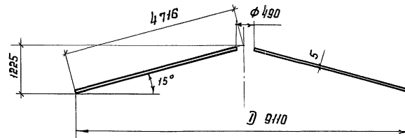
Сечение оболочки
