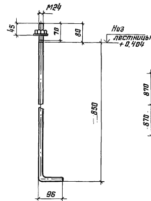
Анкерный болт
