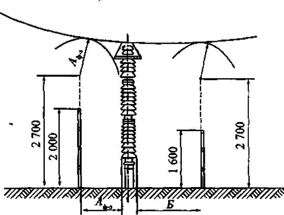
Рисунок 3 - Схема размещения оборудования. Наименьшие расстояния от токоведущих частей и элементов изоляции, находящихся под напряжением, до постоянных внутренних ограждений
