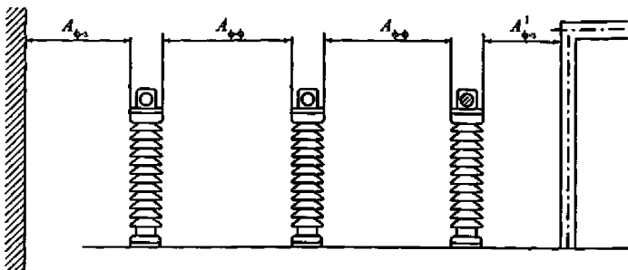
Рисунок 1 – Схема размещения оборудования. Наименьшие расстояния в свету при жестких шинах между токоведущими и заземленными частями ( A_{\Phi-З} , A'_{\Phi-З} ) и между токоведущими частями разных фаз ( A_{\Phi-Ф} )
