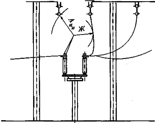
Рисунок 9 - Схема размещения оборудования. Наименьшие расстояния от подвижных контактов разъединителей в отключенном положении до заземленных и токоведущих частей
