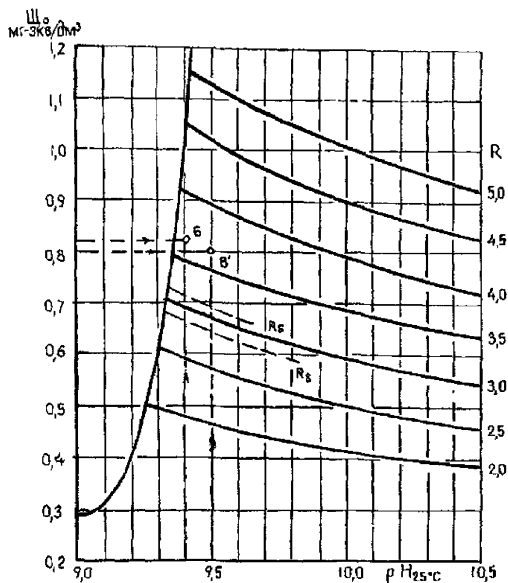
Рисунок Б.10в - Номограмма II. Зависимость щелочности от величины рН
