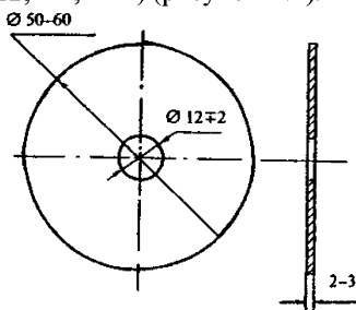
Рисунок В.1 - Пластина - индикатор коррозии
