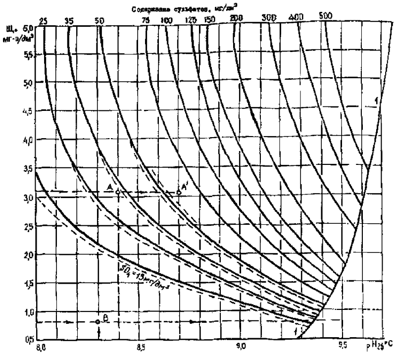
Рисунок Б.2 - Номограмма 1.1 для вод с содержанием хлоридов от 15 до 50 мг/дм 3 Примечание - Пунктиром показаны изолинии для содержания хлоридов 15 мг/дм 3 , там, где есть существенные отличия от других диапазонов.
