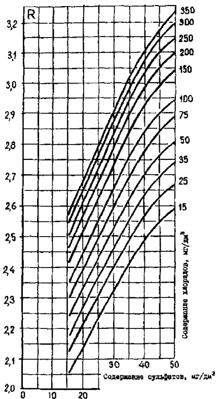
Рисунок Б.10б - Номограмма II. Определение параметра R для низких содержаний сульфатов
