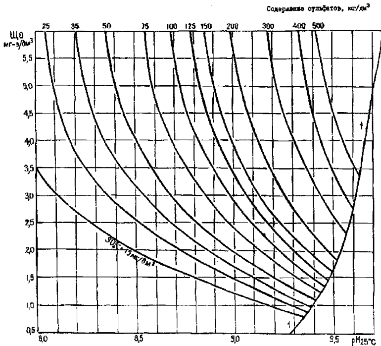
Рисунок Б.3 - Номограмма 1.2 для вод с содержанием хлоридов 75 мг/дм 3
