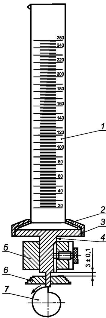
1 — мерный цилиндр; 2 — резиновая втулка; 3 — держатель для мерного цилиндра; 4 — ось; 5 — втулка; 6 — наковальня; 7 — кулачок
