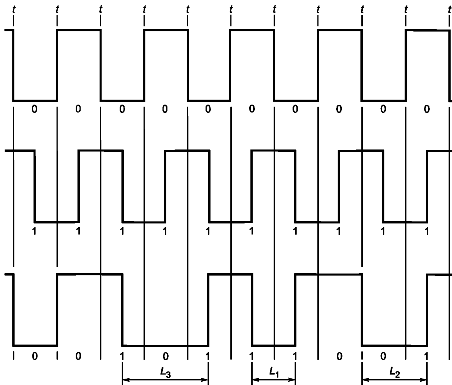
Рисунок 8 — Пример кодирования методом МЧМ
