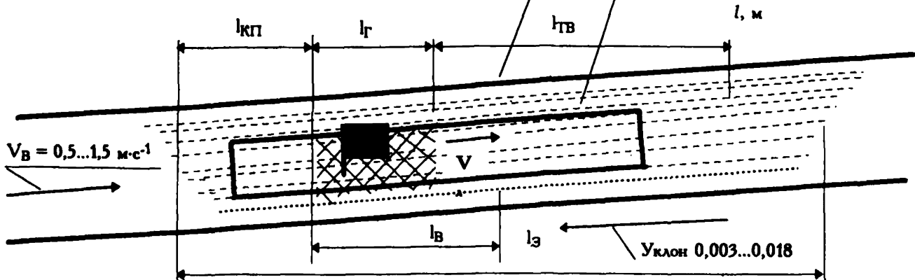
Рис. 1. Схема обстановки при развитом пожаре подвижного состава в тоннеле:
