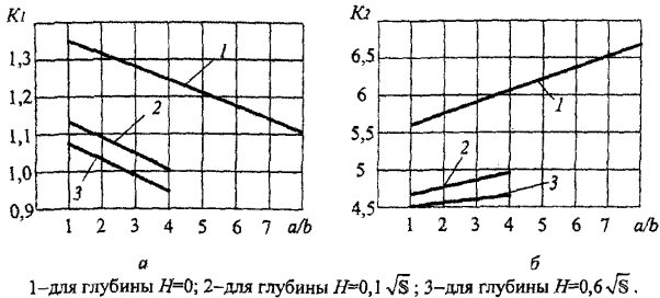
Рисунок Д.2 - Зависимости коэффициентов K_1 = f(a/b) и K_2 = f(a/b)
