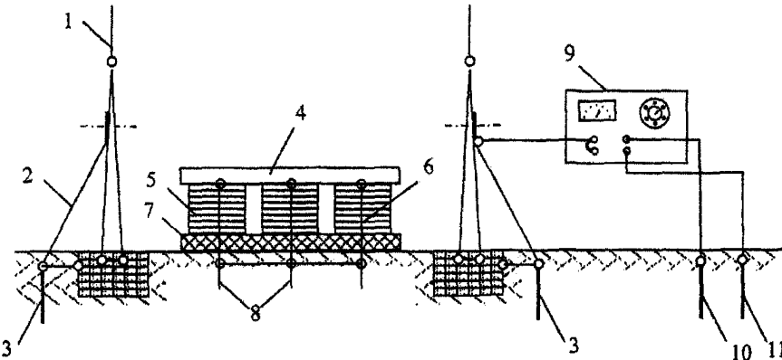
1-молниеприемник; 2-токопуск; 3-искусственный заземлитель молниеотвода; 4-металлическая крыша хранилища; 5-штабелю с изделиями; 6-заземляющие проводники металлической крыши; 7-диэлектрический фундамент хранилища; 8-электроды заземления объекта; 9-измерительный прибор; 10, 11-потенциальный и токовый электроды измерительного прибора
