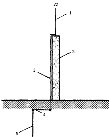
Рисунок 3.2 - Рекомендуемые варианты конструктивного решения заземлителей для стержневых молниеприемников
