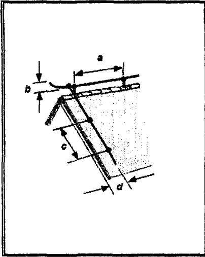
а) устройство молниеприемного проводника на коньке крыши и вертикального спуска по скату крыши
