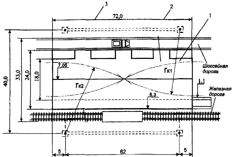
1—хранилище; 2—молниеотвод; 3—фундамент молниеотвода; 4—горизонтальный электрод заземления; 5—вагон; \Gamma_{к1} —радиус защиты молниеотвода первой линии; \Gamma_{к2} —радиус защиты молниеотвода второй линии
