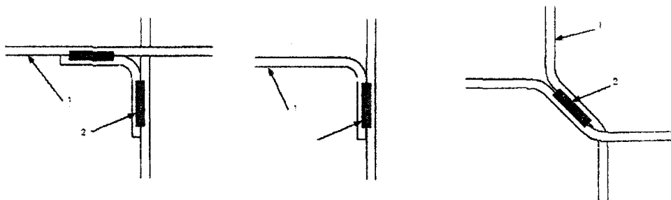
Рисунок Г.27 - Сварное соединение проводников с арматурой железобетона
