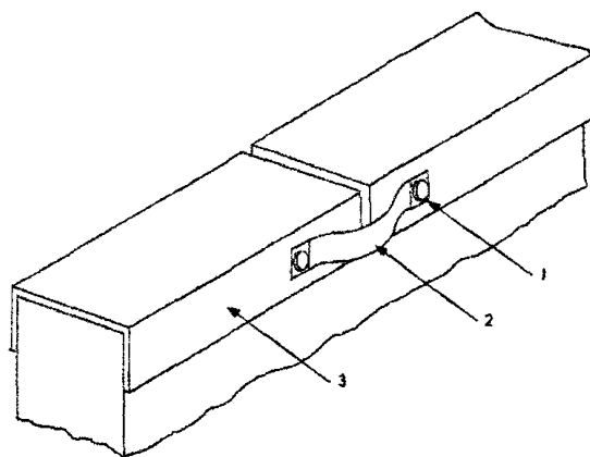
1 – коррозионно-стойкое крепление; 2 – гибкий проводник; 3 – металлическое покрытие парапета Рисунок Г.30 - Пример устройства металлического покрытия на парапете крыши
