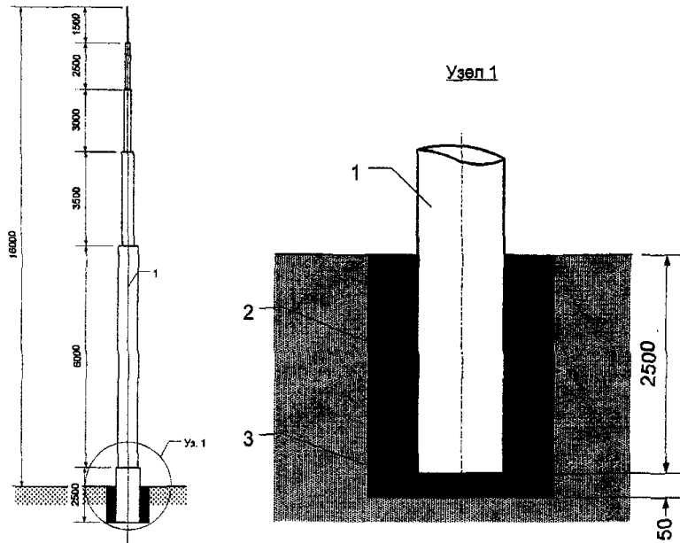
1-основание молниеотвода; 2-раствор бетона; 3-металлическая плита толщиной – 8мм
