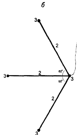
Рисунок 3.2 - Рекомендуемые варианты конструктивного решения заземлителей для стержневых молниеприемников
