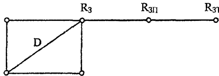
Рисунок Д.2.1 - Однолучевая схема измерений
