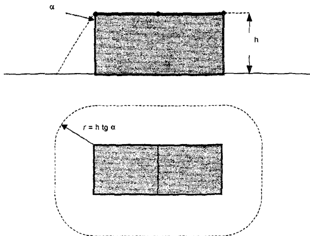
Рисунок Г.18 - Зона защиты молниеприемной сетки, установленной непосредственно на кровле здания
