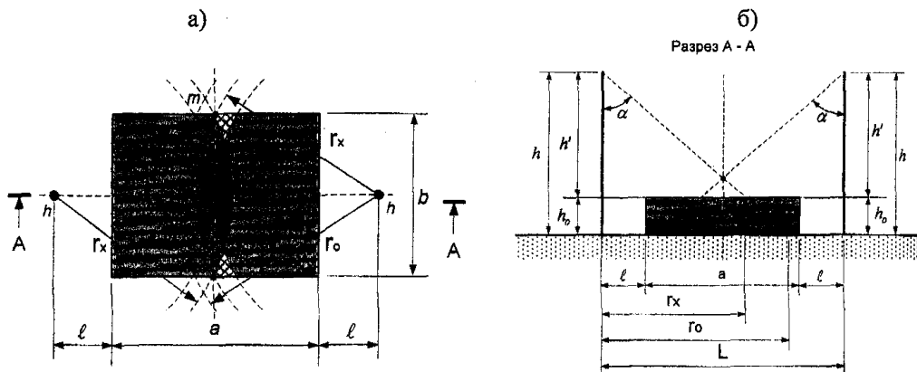
Рисунок 2.3 – Схема для расчета высоты двухстержневых молниеотводов
