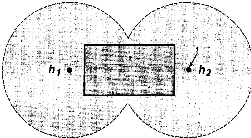
1 – молниеприемник; 2 – объект
