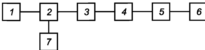
1 — измерительный генератор; 2 — фильтр; 3, 5 — коаксиальные соединители; 4 — эталонный делитель напряжения; 6 — поверяемый вольтметр; 7 — эталонный вольтметр
