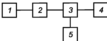
1 — измерительный генератор; 2 — фильтр; 3 — коаксиальный соединитель; 4 — поверяемый вольтметр; 5 — эталонный вольтметр
