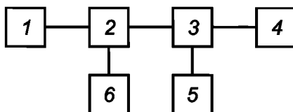
1 — измерительный генератор; 2, 3 — коаксиальный соединитель; 4 — поверяемый вольтметр; 5 — эталонный вольтметр; 6 — эталонный частотомер
