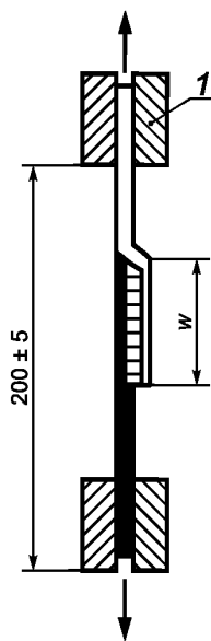
1 — зажим; w — ширина клеевого соединения
