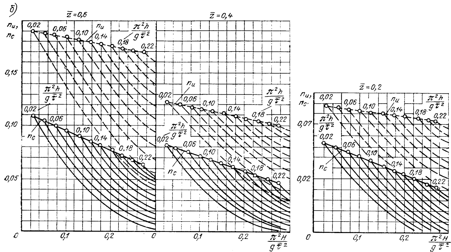
Рис. 153б. Графики значений коэффициентов \nu_u и \nu_c .
