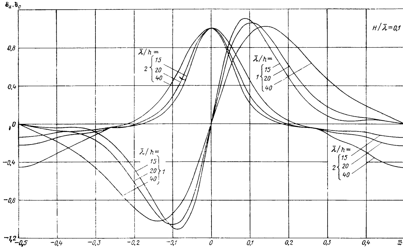
Рис. 34. Графики значений коэффициентов сочетаний инерционного \delta_i (графики 1) и скоростного \delta_c (графики 2) компонентов нагрузки от волн при H/\bar{\lambda} = 0,1 .
