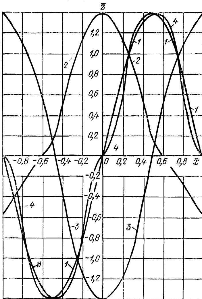
Рис. 149. Графики значений коэффициентов сочетания инерционного \delta'_{xn} (график 1), \delta'_{zn} (график 3) и скоростного \delta'_{xc} (график 2), \delta'_{zc} (график 4) компонентов горизонтальной и вертикальной нагрузки от волн.
