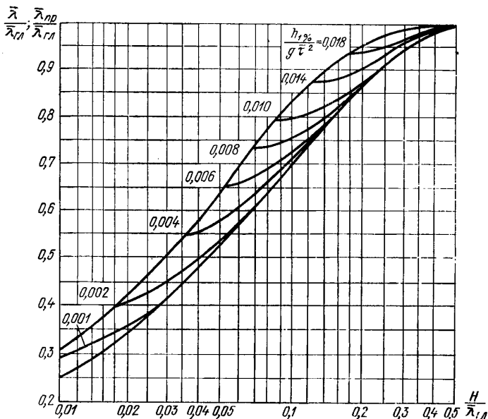
Рис. 123(41). Графики для определения значений \frac{\bar{h}_i}{\bar{\lambda}_{гд}} в мелководной и \frac{\bar{\lambda}_{пр}}{\bar{\lambda}_{гд}} в прибойной зонах.
