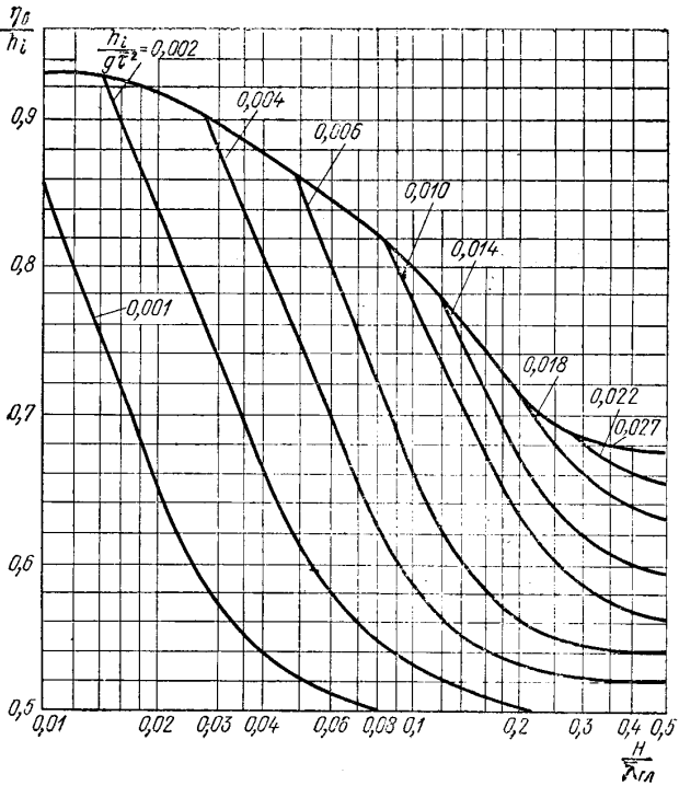
Рис. 118 (40). Графики для определения значений \frac{\eta_v}{\eta_i} .
