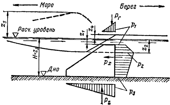
Рис. 68 (26). Эяграммы волнового давления на подводный волнолом.
