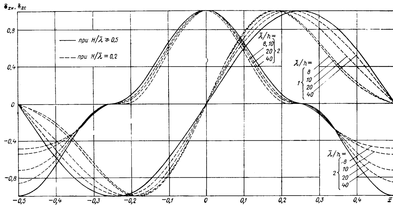
Рис. 38 (18). Графики значений коэффициентов сочетания инерционного \delta_{xи} (графики 1) и скоростного \delta_{xc} (графики 2) компонентов горизонтальной нагрузки от волн.
