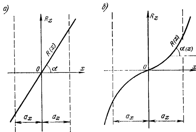
Рис. 170. Графики жестких характеристик для симметричных систем заякорения а—линейная; б—нелинейная.
