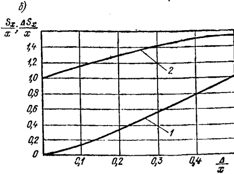
Рис. 176. График зависимости ширины площадки контакта \Delta S_x и поперечного размера деформированного отбоя S_x от относительной его деформации \Delta/x для цилиндрических отбойных устройств трубчатого сечения при отношении внутреннего и наружного диаметра 1:2
