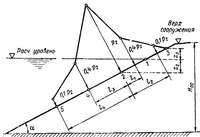
Рис. 24(11). Эюра максимального расчетного волнового давления на откос, укрепленный плитами.
