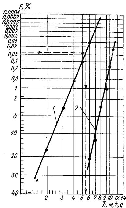
Рис. 121. Режимные функции высоты \bar{h} (1) и периода \bar{\tau} (2).
