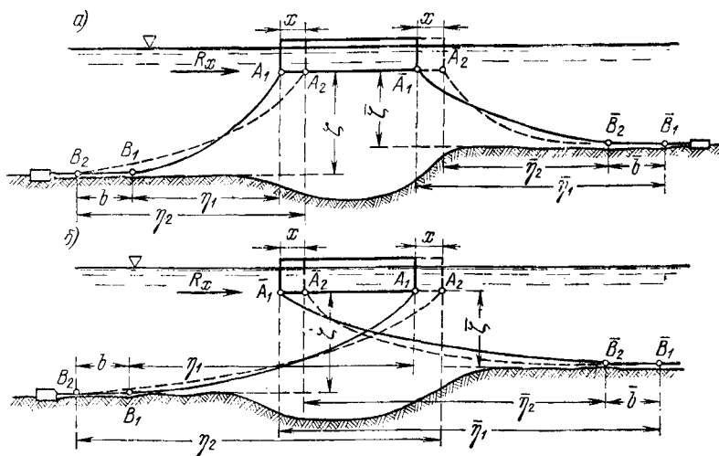
Рис. 162. Схемы раскрепления плавучих объектов цепями без подвесных грузов (длинные цепи) а — обыкновенная схема закорення; б — перекрестная схема закорення при необходимости обеспечения глубины у кордона.
