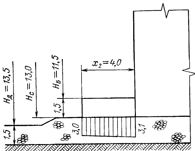
Рис. 13. Эюра взвешивающего волнового давления на берменные массивы (размеры в м, ординаты эюр в тс/м 2 ).
