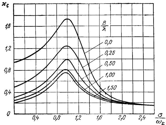
Рис. 175. График для определения величины коэффициента \kappa_c .
