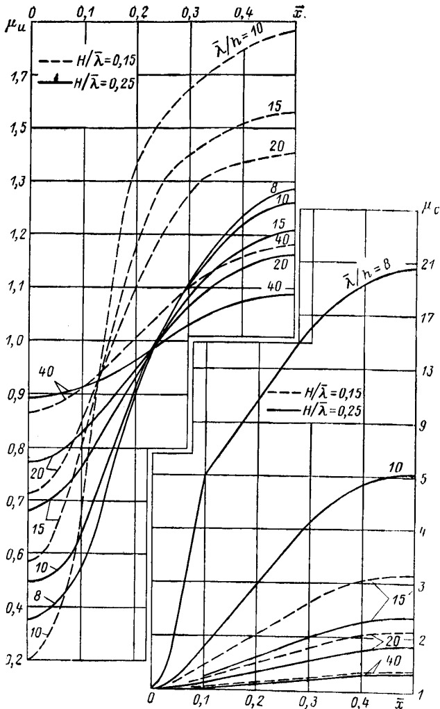
Рис. 52. Графики значений инерционного \mu_{и} и скоростного \mu_{с} коэффициентов фазы при H/\bar{\lambda} = 0,15 и 0,25 .
