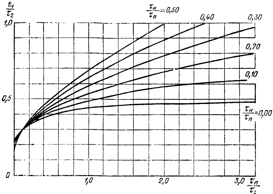
Рис. 147. График для определения значений t_1 .
