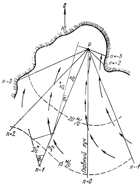
Рис. 120. Графические построения для определения элементов волн в расчетной точке P по заданному полю ветра.
