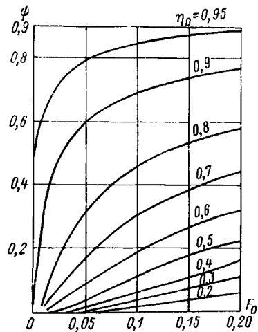
Рис. 107 (35). Графики значений коэффициента \psi .
