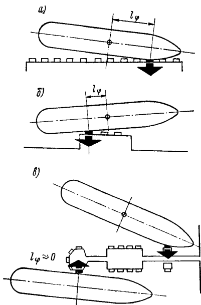
Рис. 90. Расчетные случаи навала судна на причал.
