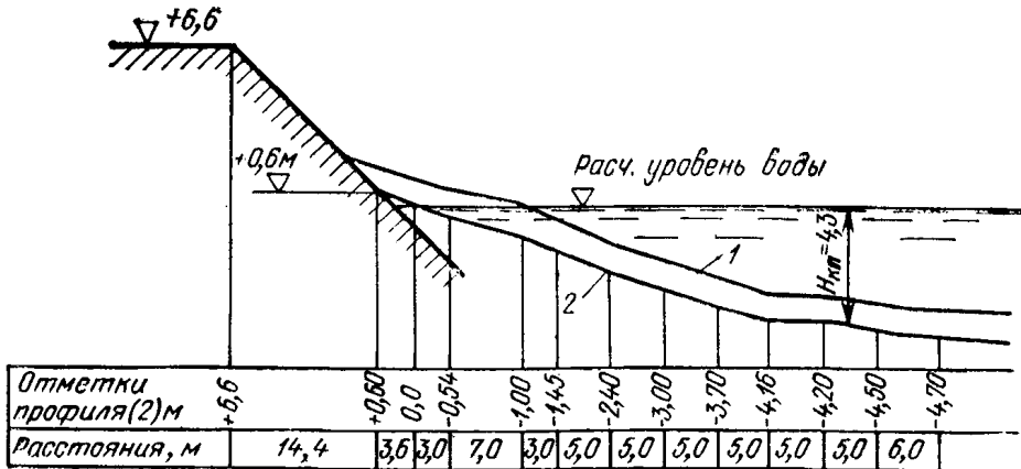
Рис. 160. Схема к расчету наката волн на откос, покрытый галечным пляжем
