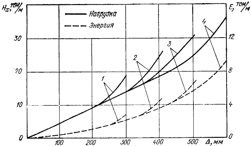
Рис. 179. График зависимостей реакций H_x и энергоемкости E цилиндрических резиновых отбойных устройств от величины деформаций \Delta для цилиндра длиной 1,0 м типа 1—D600; 2—Dc50; 3—D1000; 4—D1200.
