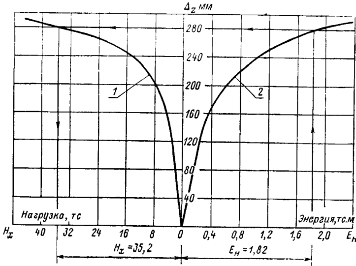
Рис. 105. Расчетные графики
