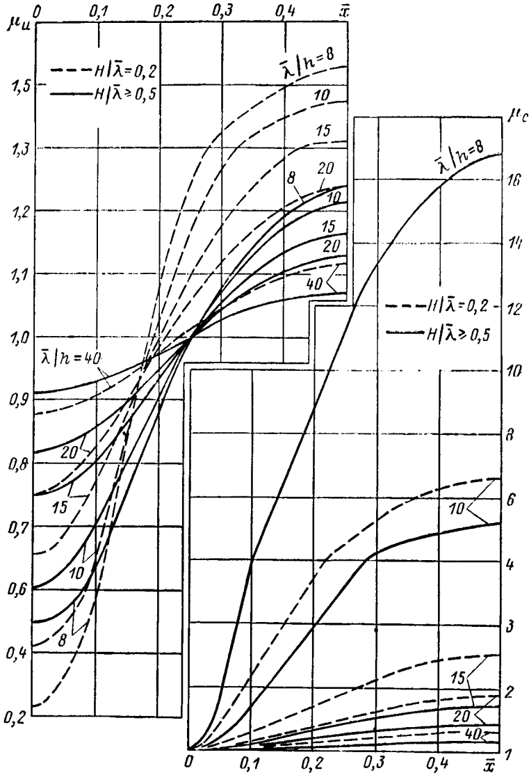
Рис. 42(22). Графики значений инерционного \mu_{in} и скоростного \mu_{cs} коэффициентов фазы.
