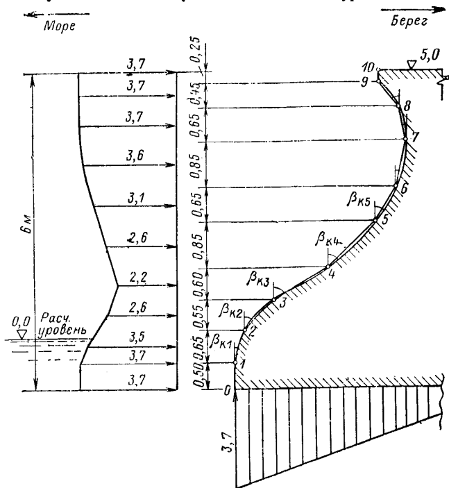
Рис. 76. Эпюры горизонтальных составляющих волнового давления на криволинейную поверхность и взвешивающего давления на постоу волноотбойной стены (ординаты эпюр в \text{тс/м}^2 ).
