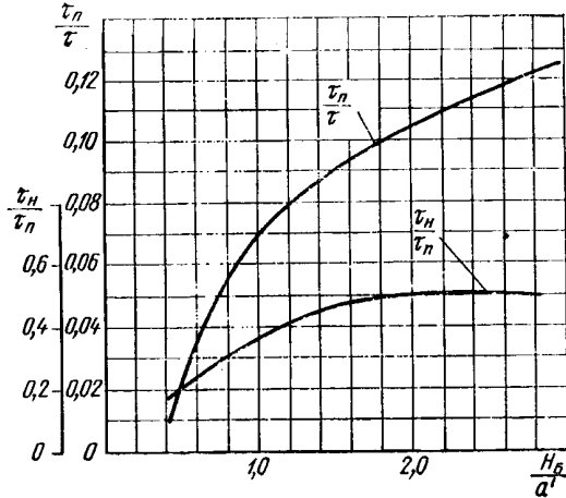
Рис. 142. Графики для определения \tau_n и \tau_{нн} .
