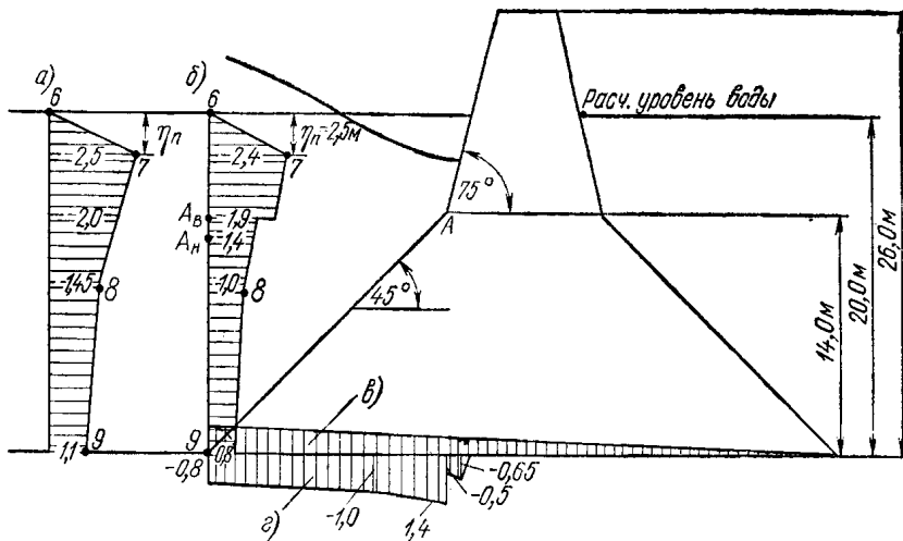
Рис. 139. Эпюры волнового давления при подходе ложбины волны а—горизонтального на вертикальную стену; б—горизонтального на крутонаклонную стену; вертикального на крутонаклонную стену (вверх); взвешивающего (вниз); ординаты давлений в тс/м 2 .
