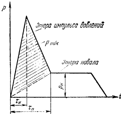
Рис. 140. Изменение нагрузок во времени при ударе волны.
