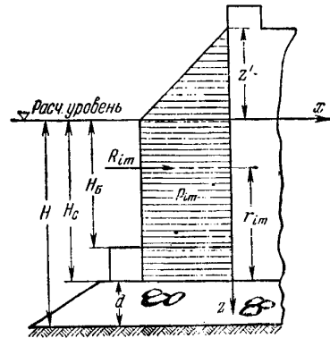
Рис. 141. Эпюра импульса давлений в момент удара волны, тс·с/м 2 .
