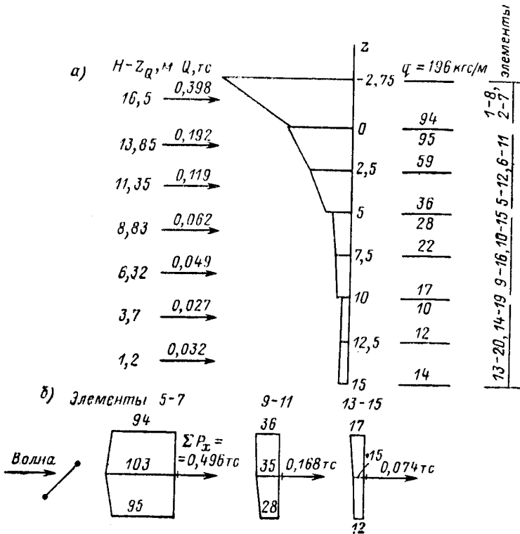
Рис. 66. Горизонтальная волновая нагрузка (к примеру 17) а — на наклонные элементы 2-7, 1-8, 6-11, 5-12, 10-15, 9-16, 14-19, 13-20; б — на горизонтальные элементы 5-7, 9-11, 13-15.
