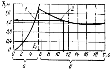
Рис. 173. Схема построения графика для определения элементов волн, предельных для стоянки пришвартованного судна у причала а — зона безопасной стоянки судна; б — безопасность судна или причала обеспечивается при ограничении элементов волн, предельных для стоянки судна.
