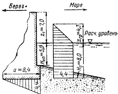
Рис. 74. Эпюры бокового и взвешивающего давлений разрушившихся волн на волноотбойную стену (размеры в м, ординаты эпюр в тс/м 2 ).
