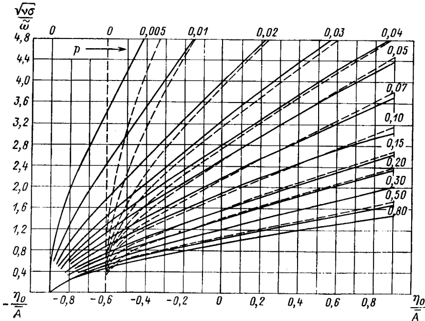
Рис. 83. График для определения параметра \frac{\eta_0}{A} сплошные линии—швартовы из синтетических и растительных материалов; пунктирные—стальные швартовы.
