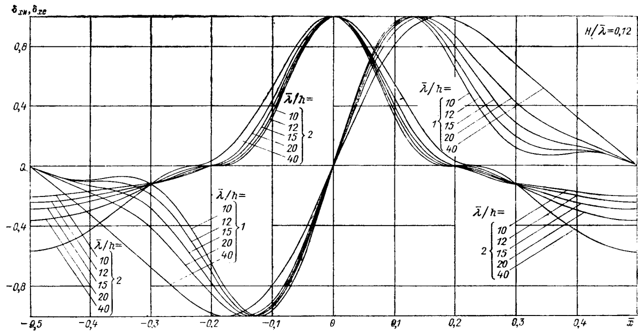
Рис. 45. Графики значений коэффициентов сочетания инерционного \delta_{xи} (графики 1) и скоростного \delta_{xc} (графики 2) компонентов удельной горизонтальной нагрузки от волн при H/\bar{\lambda} = 0,12 .
