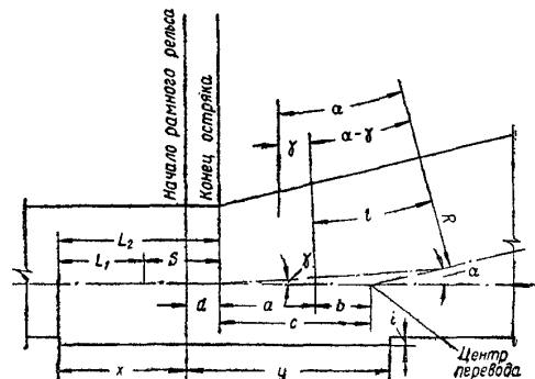
Схема для расчета длины и величины уширенной части в сопряжениях выработок
