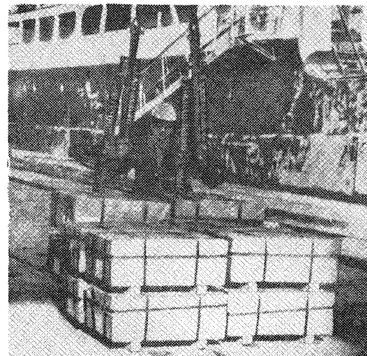
Рис. 1108.4. Установка "подъема" на причале краном, оснащенным двумя (спаренными) уравновешенными вилочными захватами. Порт Находка
