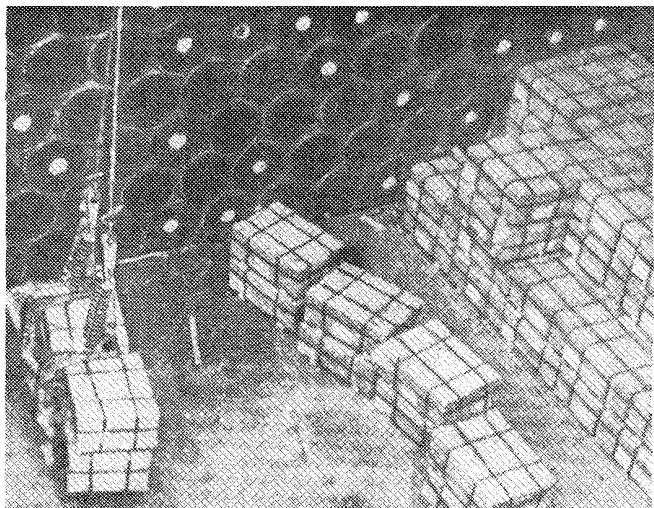
Рис. 1108.2. Выгрузка из трюма пачек металла краном, оснащенным уравновешенным вилочным захватом. Порт Находка
