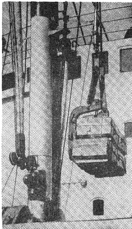
Рис. 1108.3. Выгрузка из трюма пачек металла краном, оснащенным уравновешенным вилочным захватом. Порт Находка
