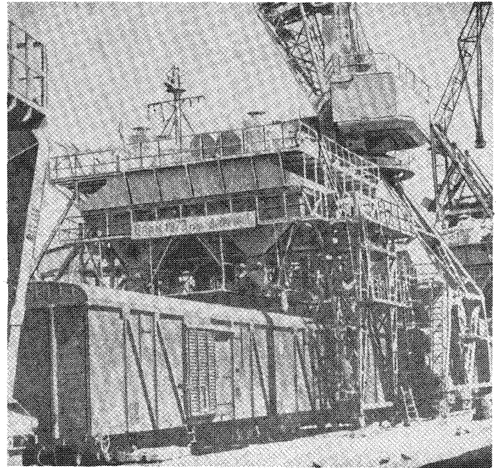
Рис. 140Г.2. Размещение пневмоперегрузателей на специальной эстакаде над бункерами. Порт Одесса
