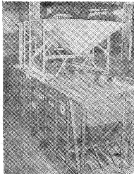
Рис. 1402.5. Установка бункера на вагон-хошер Порт Новороссийск
