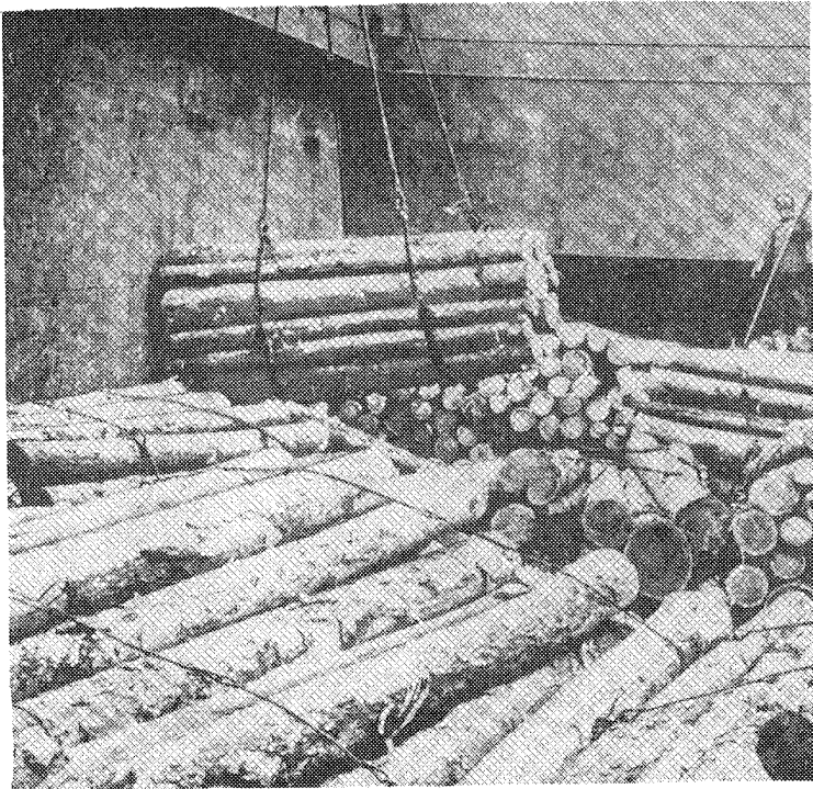
Рис. 1201.7. Формирование в просвете ложа штабеля пакетов круглого леса в полужестких стропях. Порт Ванино
