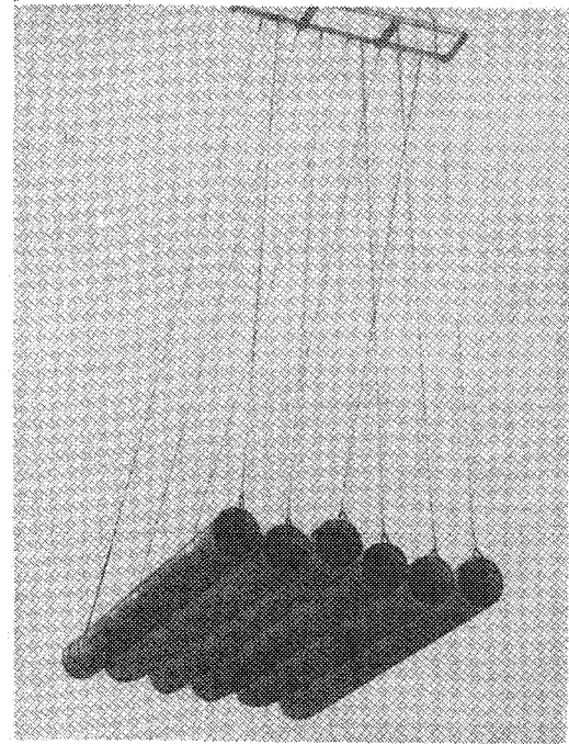
Рис. 1119.3. Перегрузка труб с помощью крана, оснащенного комплектом торцевых захватов, навешенных на раму. Порт Клай- педа
