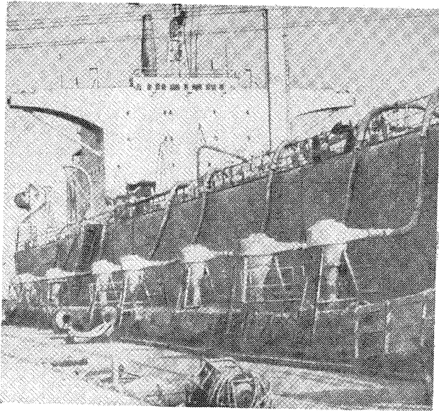
Рис. 140Г.1. Размещение пневмоперегрузателей на причале. Порт Одесса
