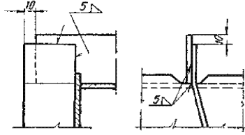
Ребра жесткости из угловой стали
