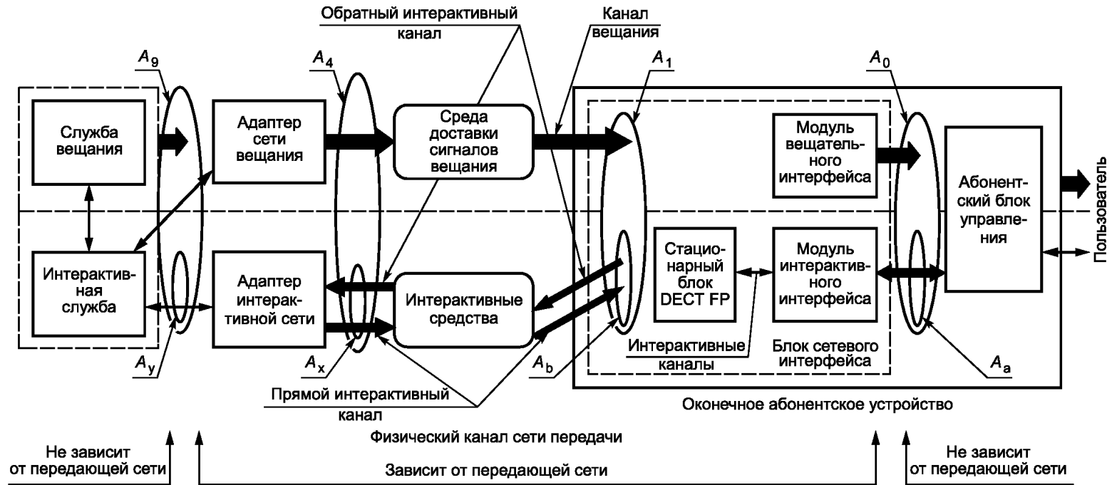
Рисунок 12 — Структурная схема функциональной модели интерактивной сети
