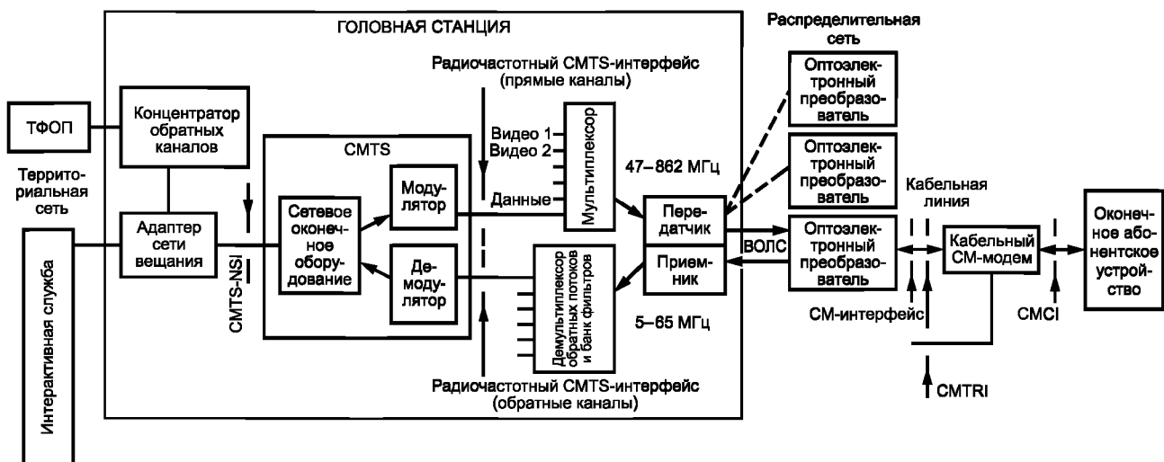
Рисунок 11 — Структурная схема интерактивной системы КТВ J.122
