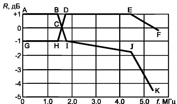
Рисунок В.1 — Шаблон допустимых значений сквозной АЧХ канала изображения по стандарту D/K (SECAM)
