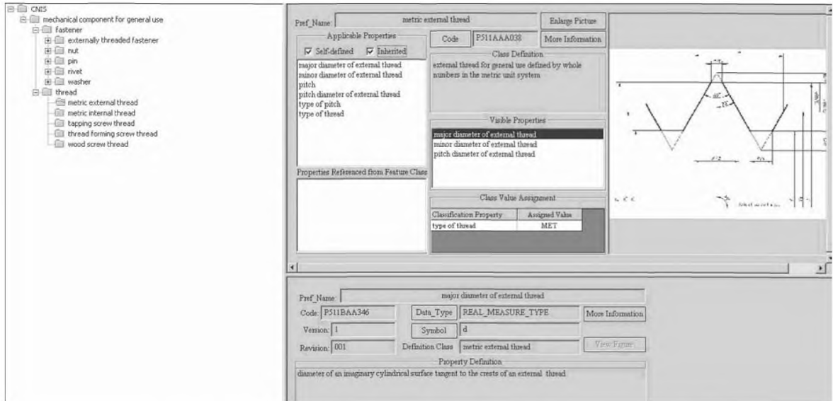
Рисунок 4 — Характеристический класс резьб по ИСО 13584-511
