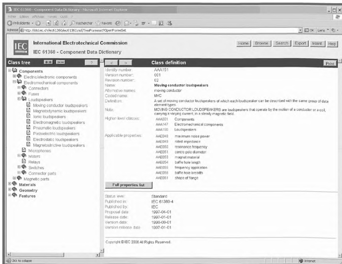
Рисунок 1 — Онлайнная база данных МЭК 61360-4-DB
