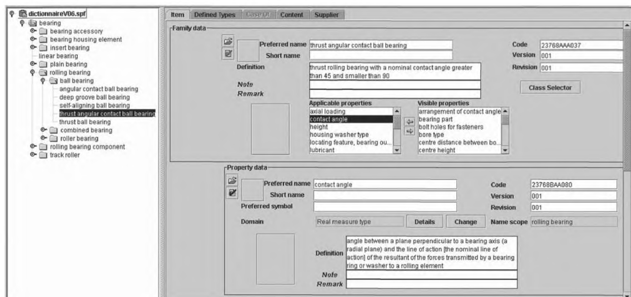
Рисунок 2 — Структура глоссария
